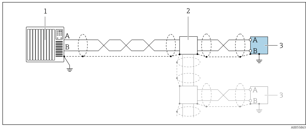
17 Anschlussbeispiel für Modbus RS485
