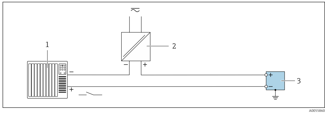
16 Anschlussbeispiel für Statuseingang
