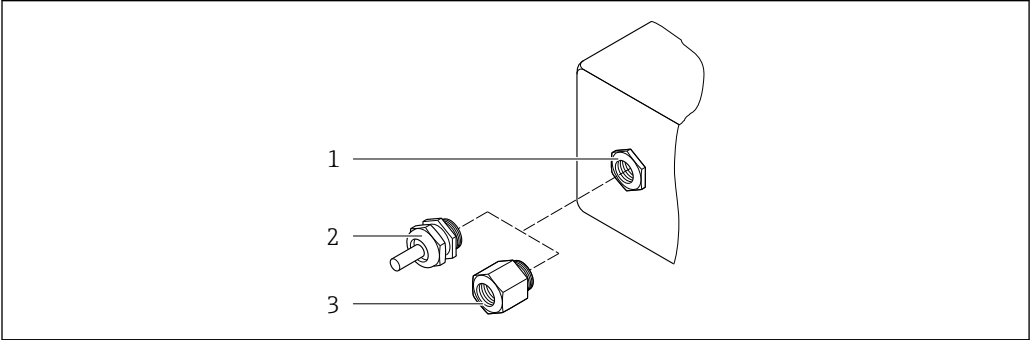
33 Mögliche Kabeleinführungen/-verschraubungen
