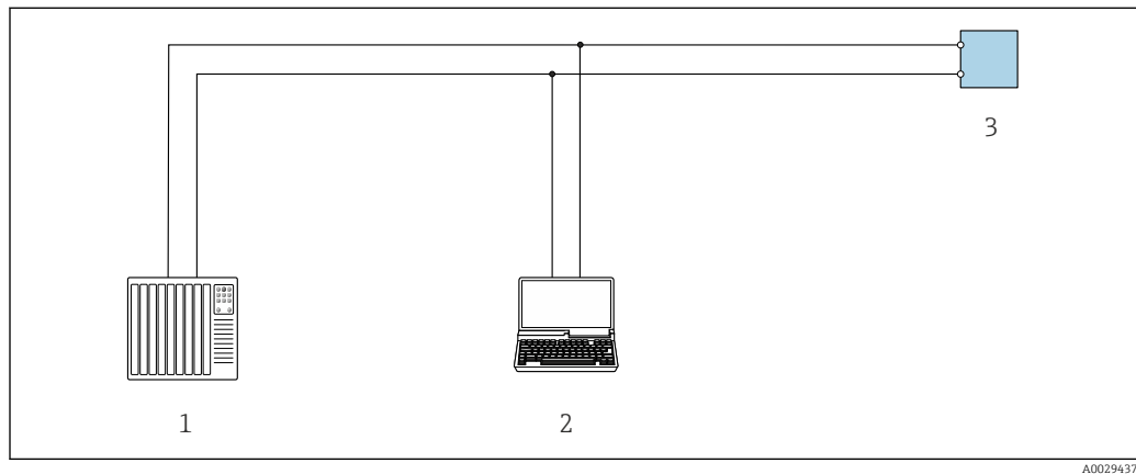
23 Möglichkeiten der Fernbedienung via Modbus-RS485-Protokoll (aktiv)
