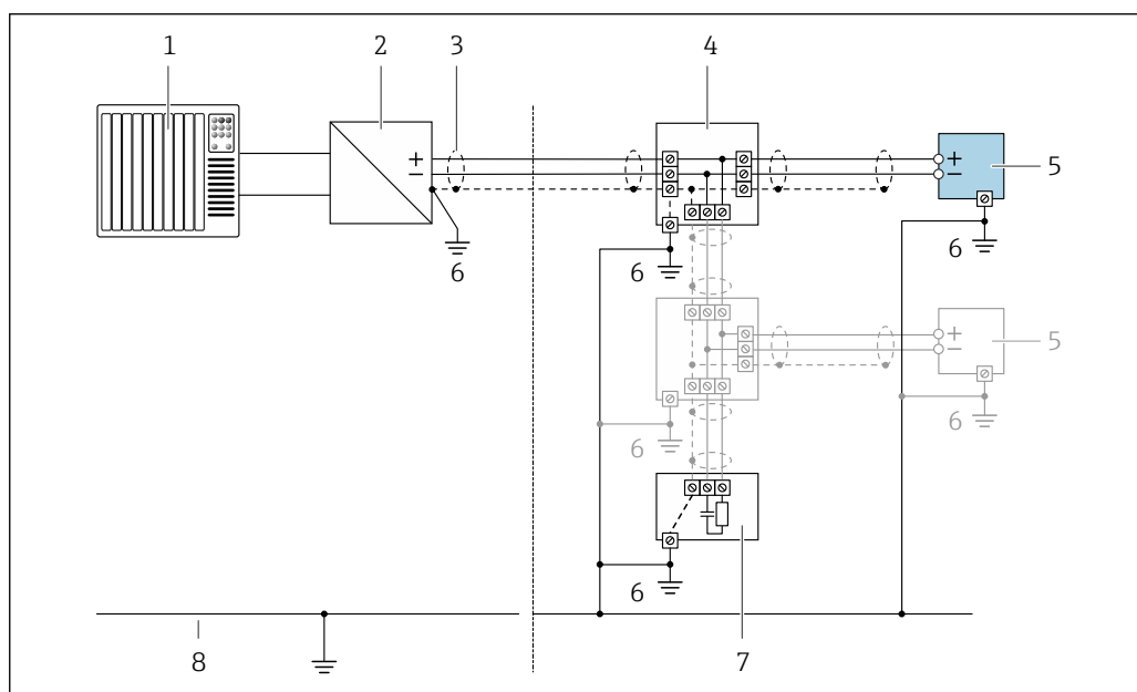
18 Пример подключения для интерфейса FOUNDATION Fieldbus
