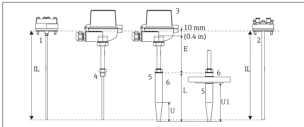
図 2 温度計の構成
