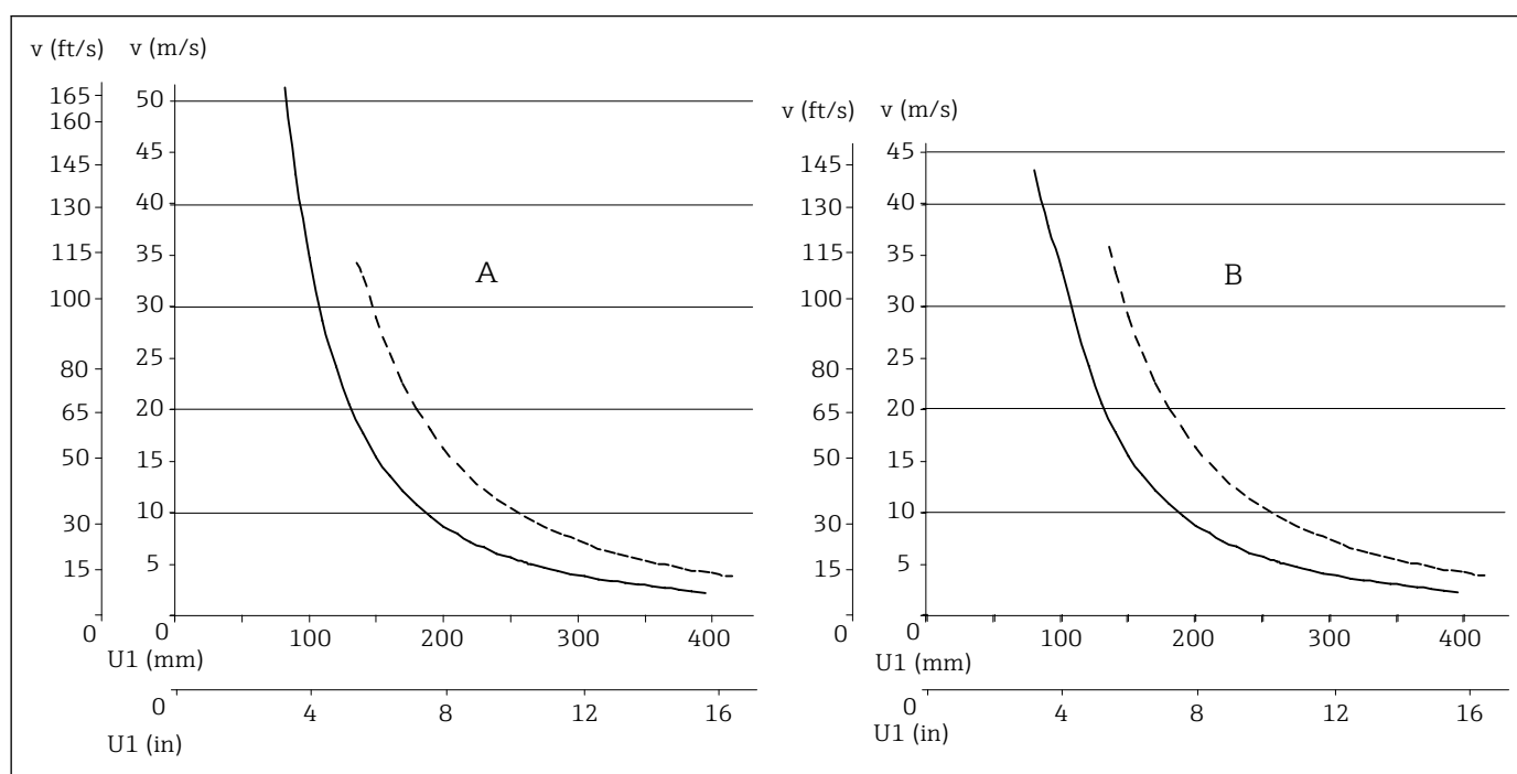
図 8 挿入長に応じた許容流速
