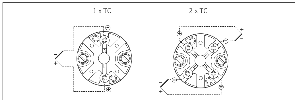
図 7 端子台
