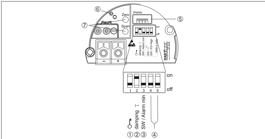
Fig. 5: Electronique HART
