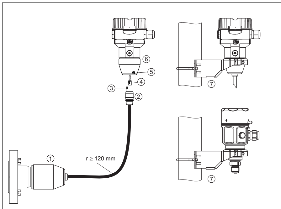
Fig. 3: Variante "Boîtier séparé"
