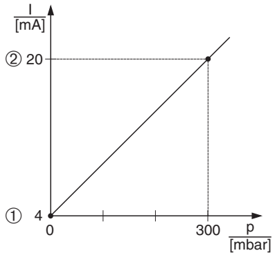
Fig. 7: Etalonnage avec pression de référence PO1-xxxxxxx-05-xx-xx-xx-010 1 voir tableau, pas 4. 2 voir tableau, pas 5.
