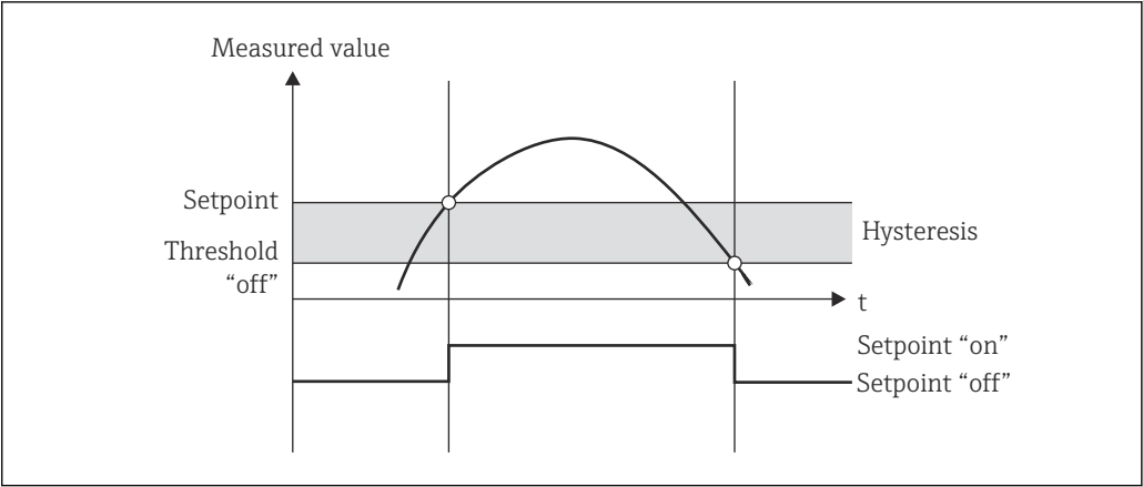
图 8 Max 工作模式
