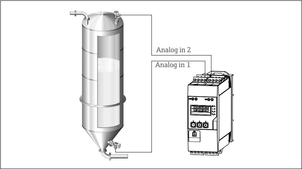
图 6 差压应用
