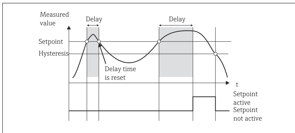
图 12 回差和延迟时间启用
