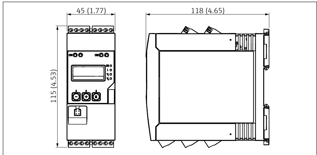
图 16 过程测控仪的外形尺寸示意图；单位：mm (in)
