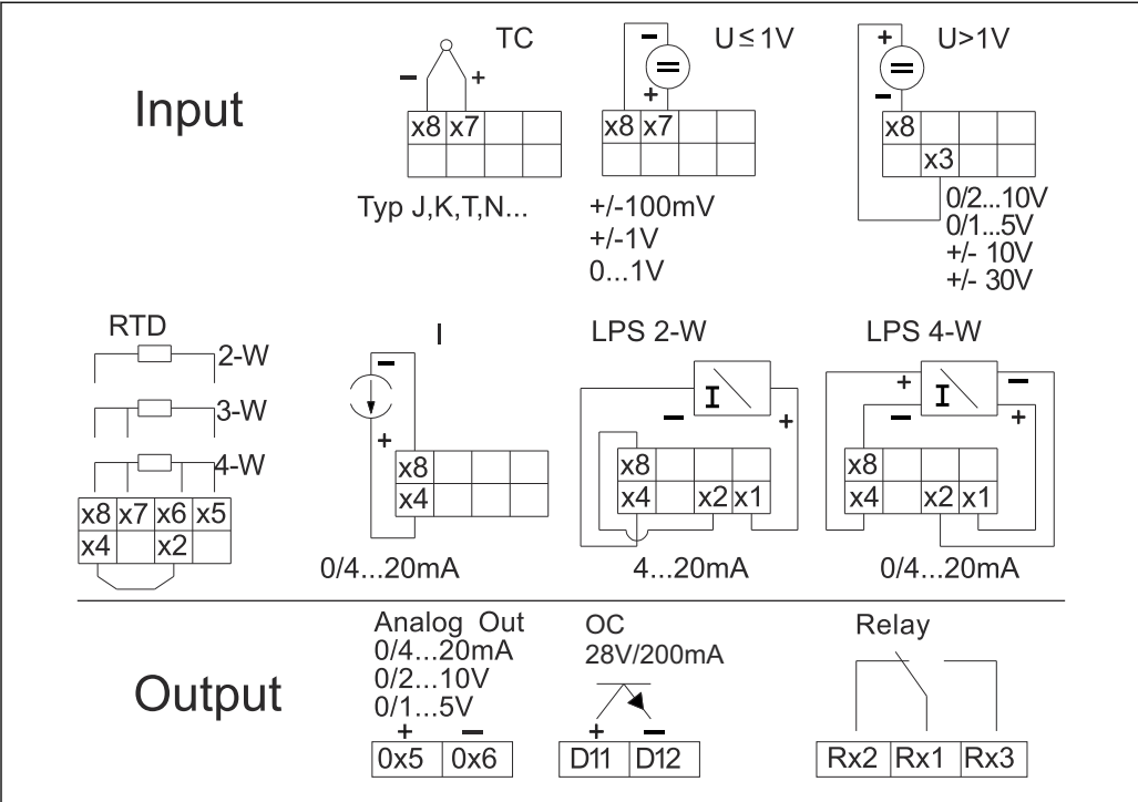
15 过程测控仪的接线端子分配（继电器（接线端子 Rx1...Rx3）和通道 2（接线端子 21...28 和 025/026），可选）；注：图示为发生电源故障时的继电器触点位置。
