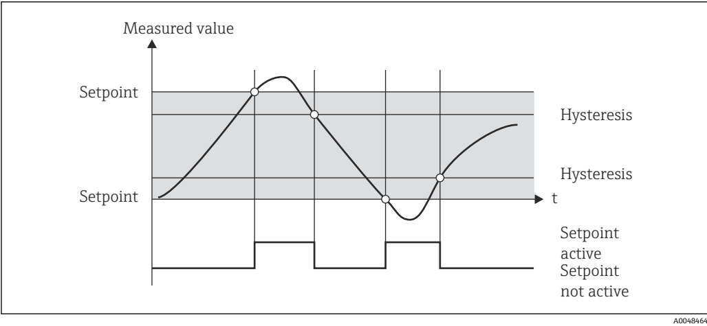
图 11 InBand 工作模式
