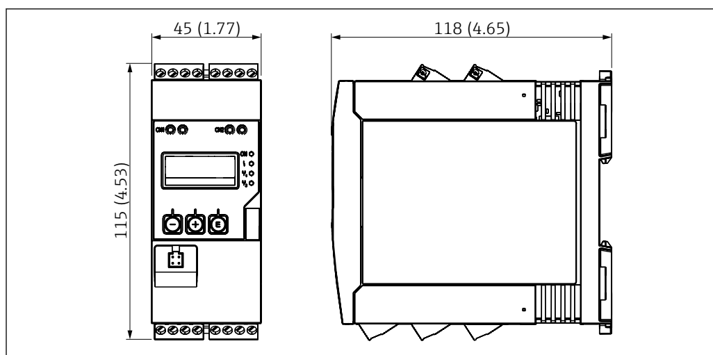
图 1 过程测控仪的外形尺寸示意图；单位：mm (in)
