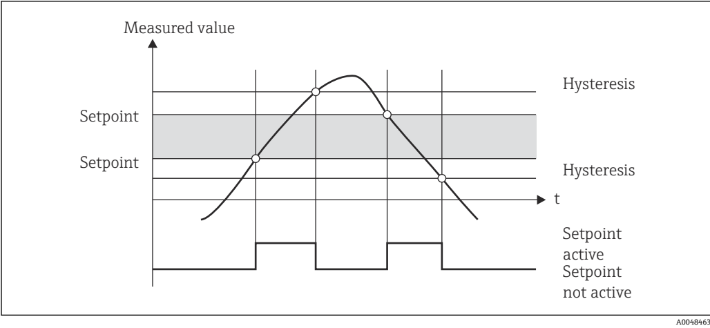
图 10 OutBand 工作模式
