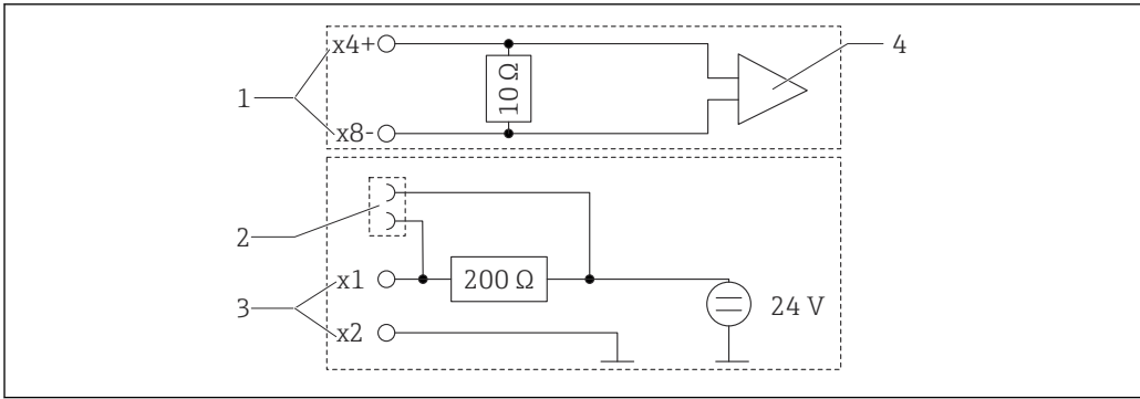
图 3 HART®连接插座的内部电路
