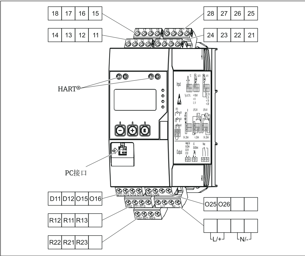
图 2 过程测控仪的接线端子分配（通道 2 和继电器，可选）
