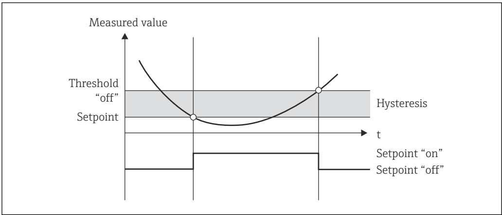
7 最小值工作模式
