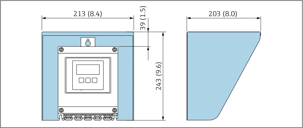
36 Tampa de proteção contra tempo para Proline 500 - digital; unidade mm (pol.)
