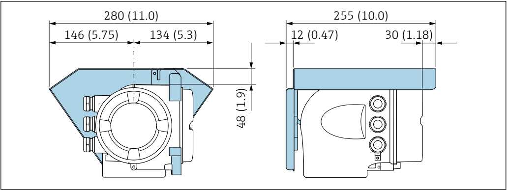
43 Tampa de proteção contra tempo para Proline 500 - unidade mm (pol.)
