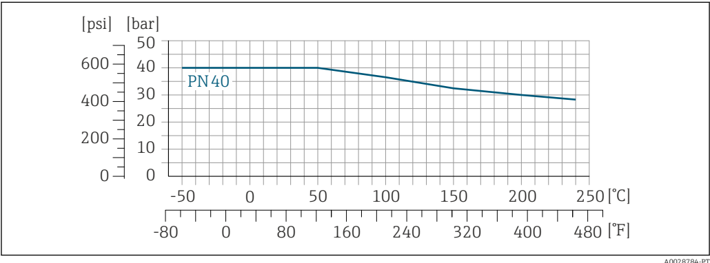
25 Com material do flange 1.4301 (F304), partes úmidas Liga C22
