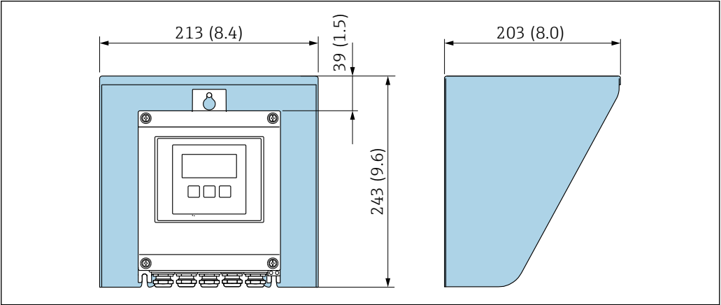
42 Tampa de proteção contra tempo para Proline 500 - digital; unidade mm (pol.)
