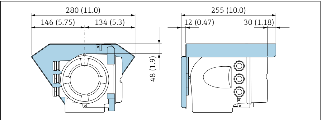
37 Tampa de proteção contra tempo para Proline 500 - unidade mm (pol.)
