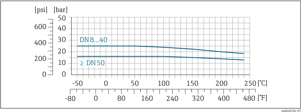
24 Com material da conexão: 1.4404 (316/316L)
