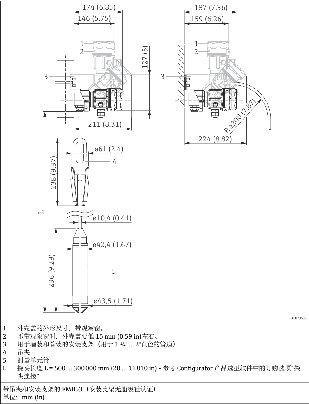
FMB53 的外形尺寸，带 F15 外壳、吊夹和安装支架
