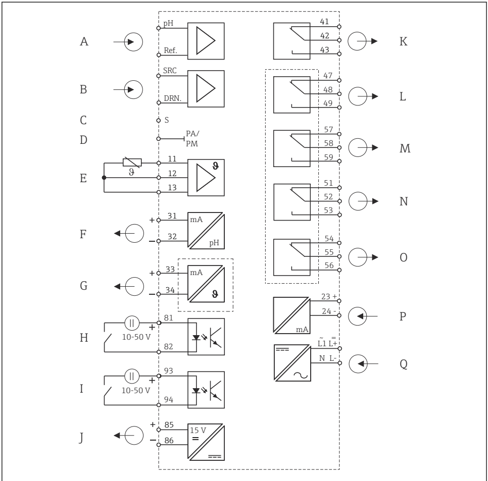
7 Elektrischer Anschluss von Messumformers ohne Memosens-Funktionalität
