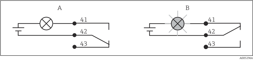
12 Empfohlene Fail-Safe-Schaltung für den Alarmkontakt
