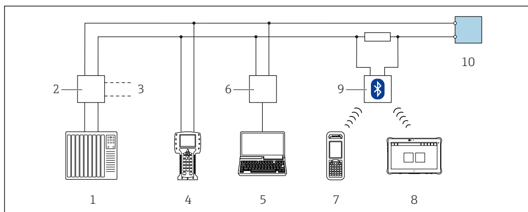
図 48 HART プロトコル経由のリモート操作用オプション（パッシブ）
