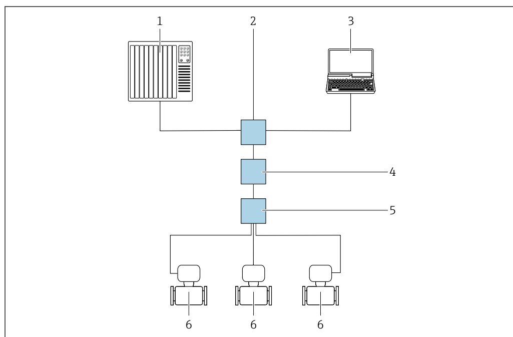
図 57 Modbus TCP over Ethernet-APL プロトコル経由のリモート操作オプション (アクティブ)
