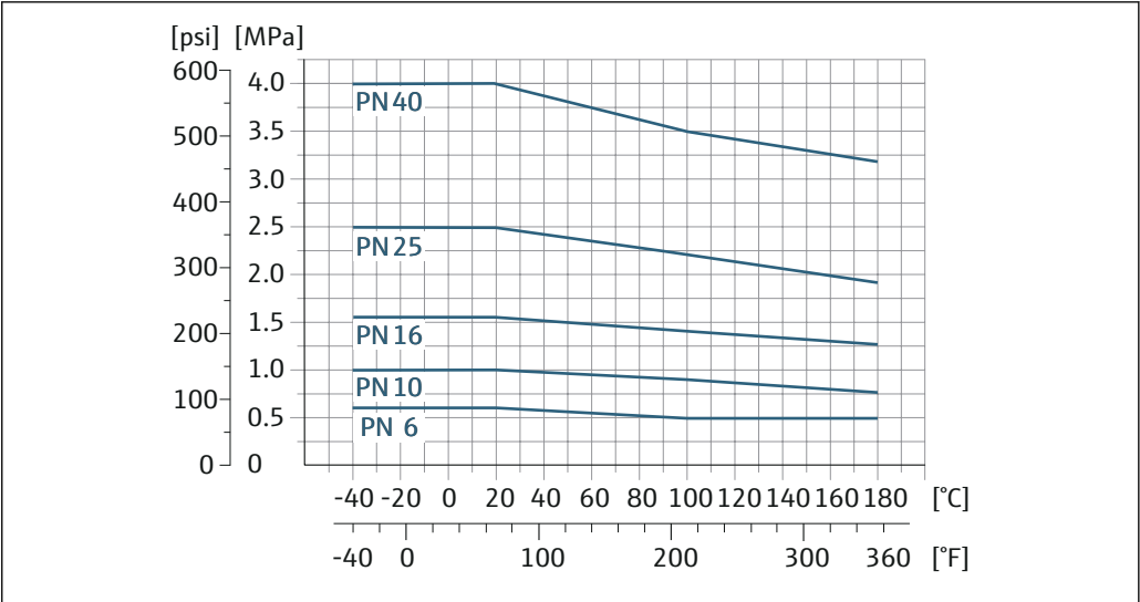
27 プロセス接続材質：ステンレス 1.4571
