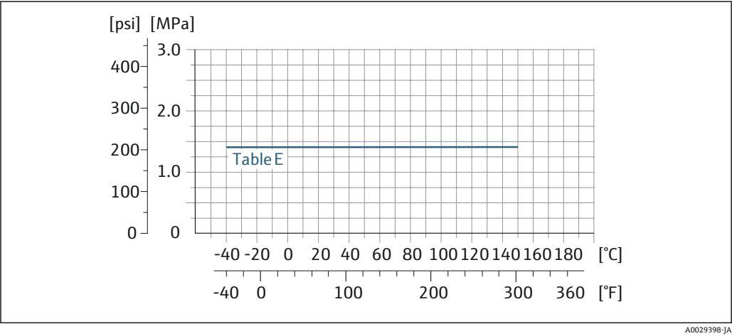
図 31 プロセス接続材質：炭素鋼 A105/S235JRG2/S275JR
