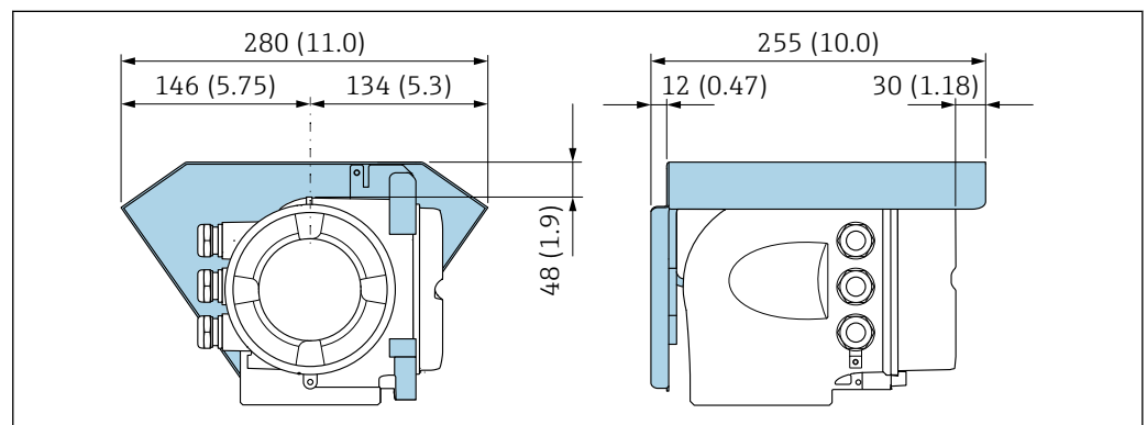
40 Proline 500 用保護カバー；単位 mm (in)
