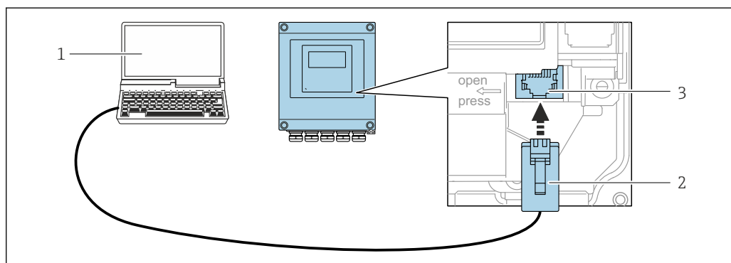
図 59 サービスインタフェース (CDI-RJ45) 経由の接続
