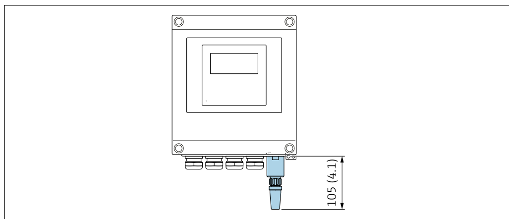
図 41 単位 mm (in)
