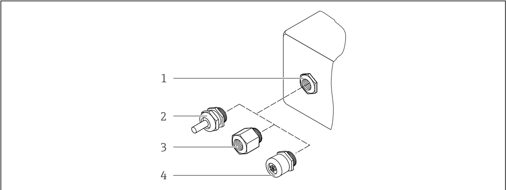
図 45 可能な電線口/ケーブルグランド
