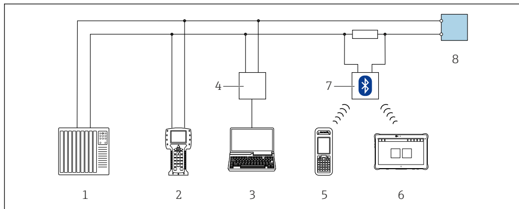
図 47 HART プロトコル経由のリモート操作用オプション（アクティブ）
