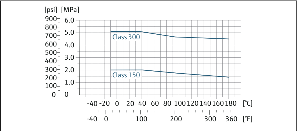
28 プロセス接続材質：炭素鋼 A105
