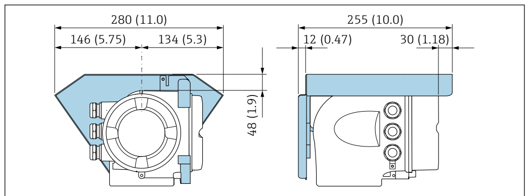
34 Proline 500 用保護カバー；単位 mm (in)
