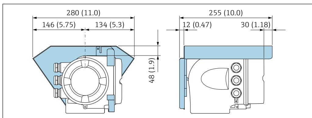
図 23 Proline 500 用保護カバー；単位 mm (in)
