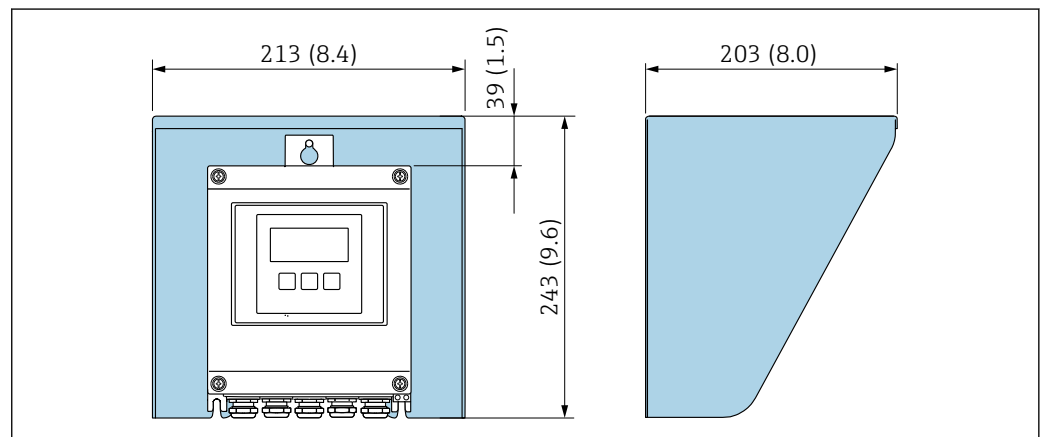
39 Proline 500 – デジタル用の保護カバー、単位 mm (in)
