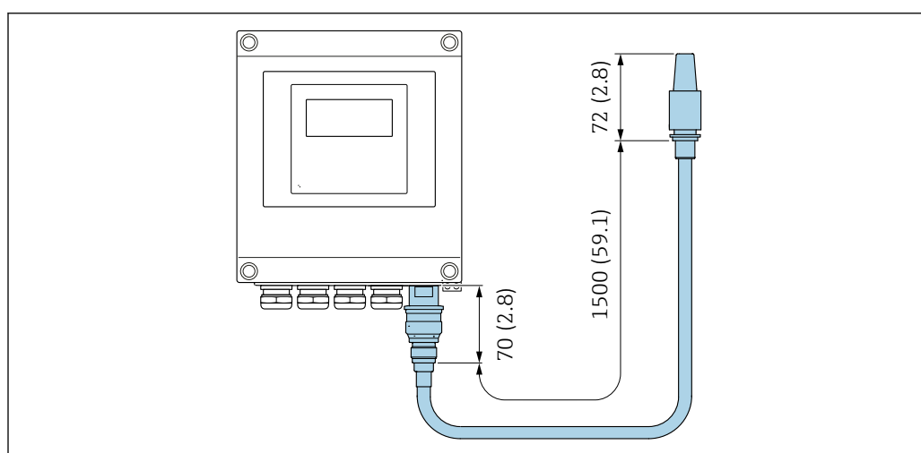
図 42 単位 mm (in)
