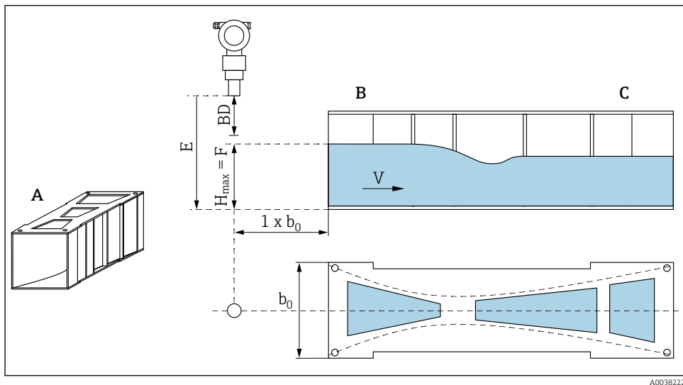
2 Лоток Хафаги-Вентури (пример)
