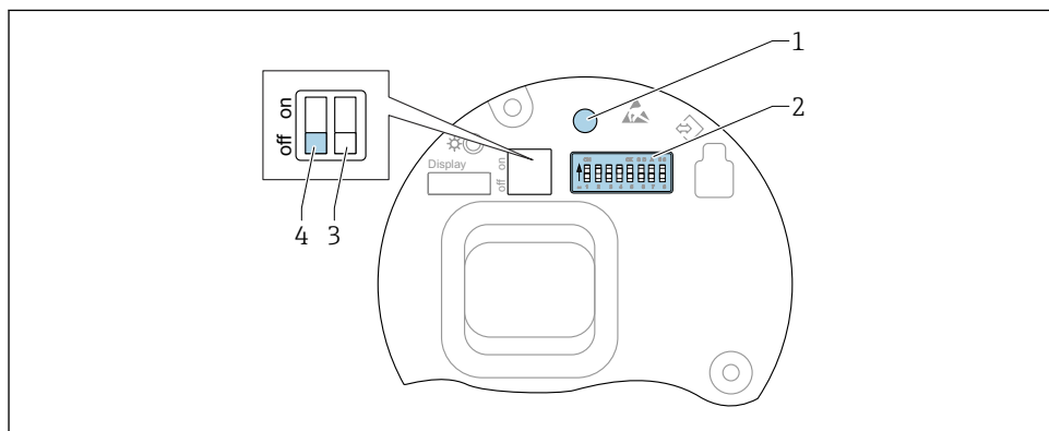
6 Teclas de configuración y microinterruptores en el módulo del sistema electrónico PROFIBUS PA
