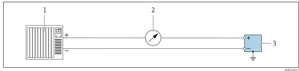
18 Exemple de raccordement pour sortie courant 4 ... 20 mA (active)
