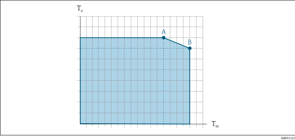
図 40 例示、値は下表を参照 Ta 周囲温度 Tm 測定物温度 A 許容最高測定物温度 Tm、Ta max = 60 °C (140 °F) 時；測定物温度 Tm が高い場合は、周囲温度 Ta を下げる必要があります。 B 規定されたセンサの最高測定物温度 Tm における許容最高周囲温度 Ta
