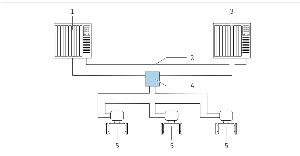
33 Пример компоновки резервируемой системы (S2): кольцевая топология
