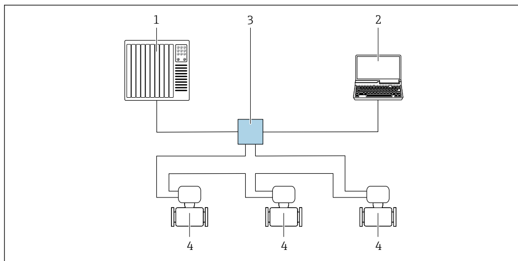
30 Варианты дистанционного управления через сеть PROFINET: топология «кольцо»
