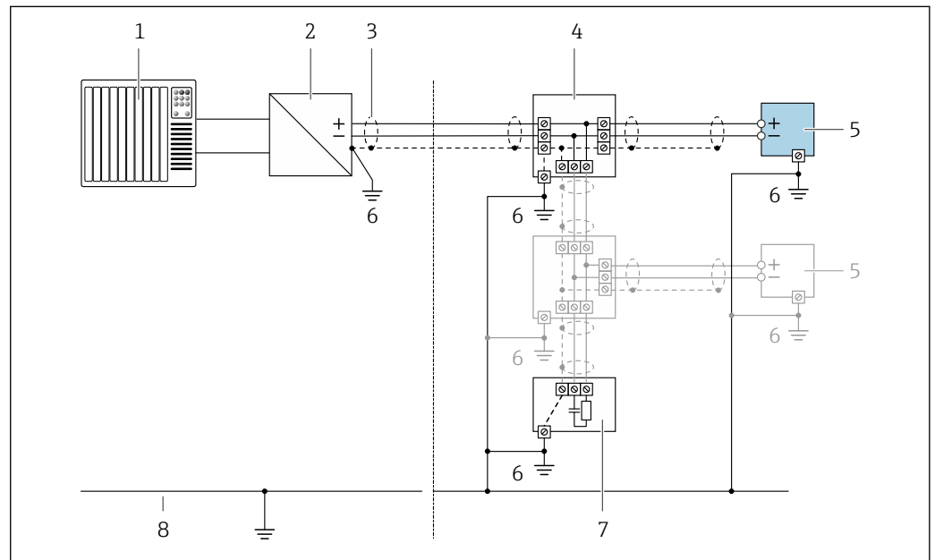
15 Esempio di collegamento per PROFIBUS PA
