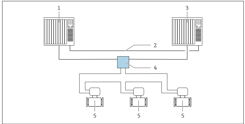
28 Exemplo do layout de um sistema redundante (S2): topologia anelar
