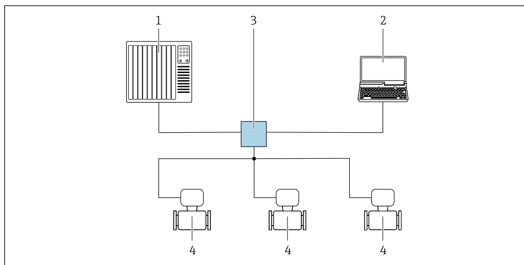
25 Opções para operação remota através da rede PROFIBUS: topologia estrela
