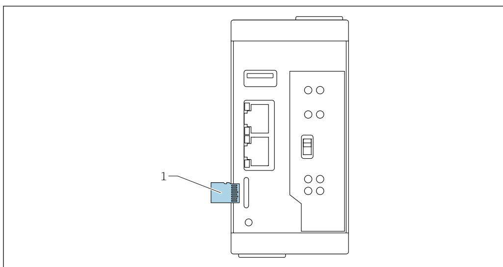
1 MicroSD 卡
