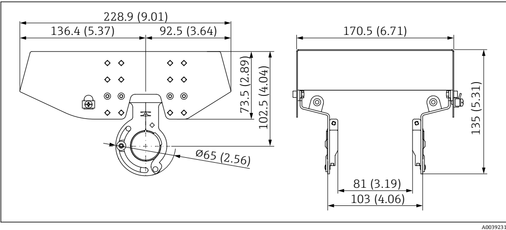
图 28 316L 防护罩 XW112 的外形尺寸示意图。测量单位 mm (in)
