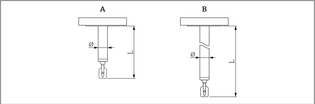
18 探头类型: 短管型, 延长管型。测量单位 mm (in)
