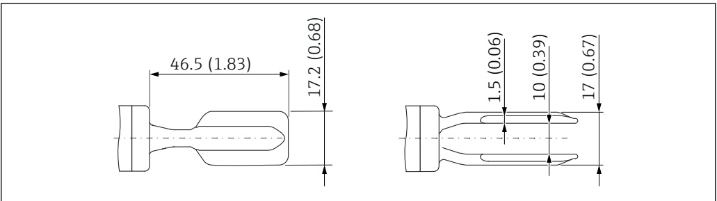
20 音叉, 带搪瓷涂层。测量单位 mm (in)
