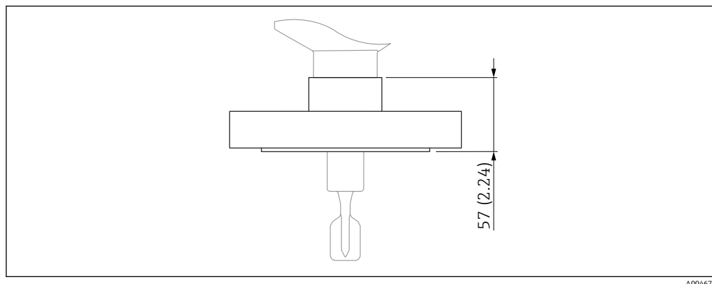
图 21 法兰过程连接（最大高度规格）。测量单位 mm (in)
