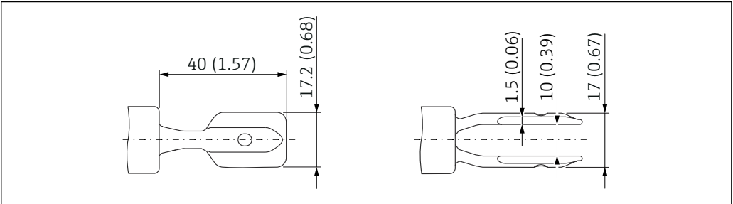
19 音叉, 带塑料涂层 (ECTFE、PFA)。测量单位 mm (in)
