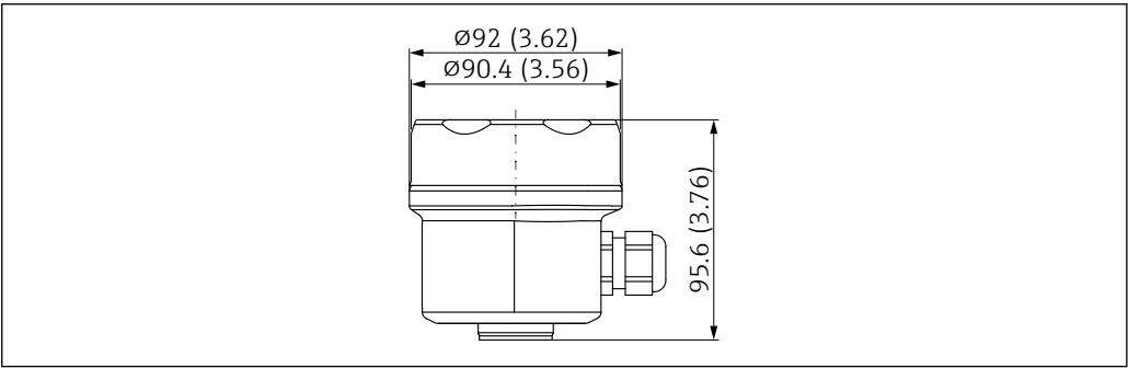
16 单腔体 316L 外壳（卫生型）的外形尺寸示意图；外壳盖不带观察窗。测量单位 mm (in)
