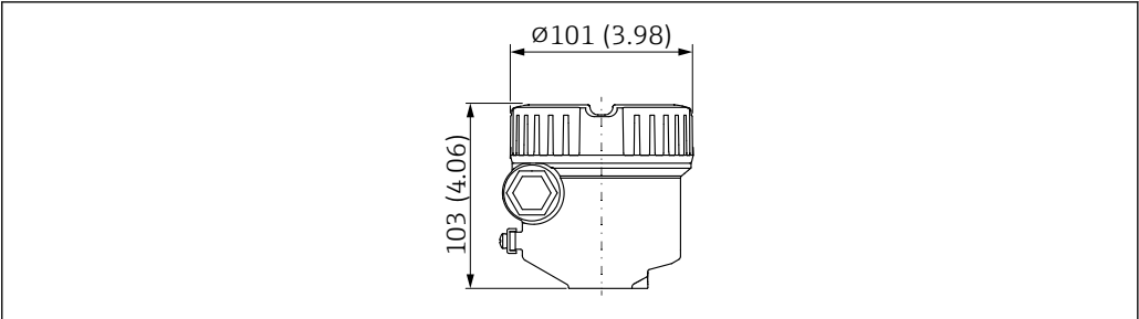
14 单腔体铝外壳的外形尺寸示意图；外壳盖不带观察窗。测量单位 mm (in)
