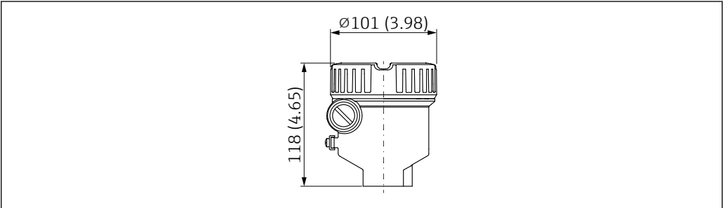
15 单腔体铝外壳（带涂层）的外形尺寸示意图；适用 Ex d/XP、粉尘防爆场合；外壳盖不带观察窗。测量单位 mm (in)
