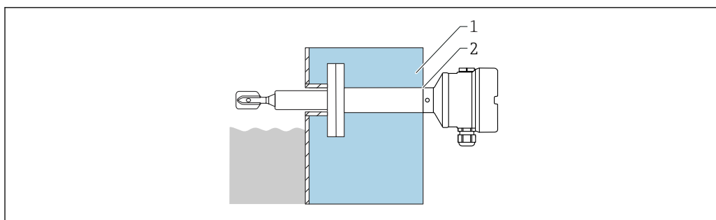
图 10 实例：带保温层的罐体
