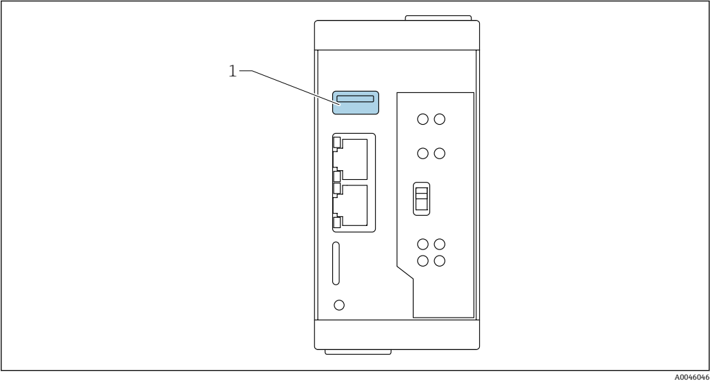
图 27 USB 接口位置
