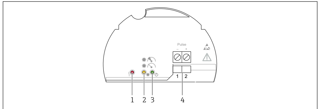
图 21 电子插件 FEL60D
