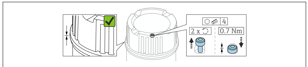
图 18 带锁定螺丝的外壳盖
