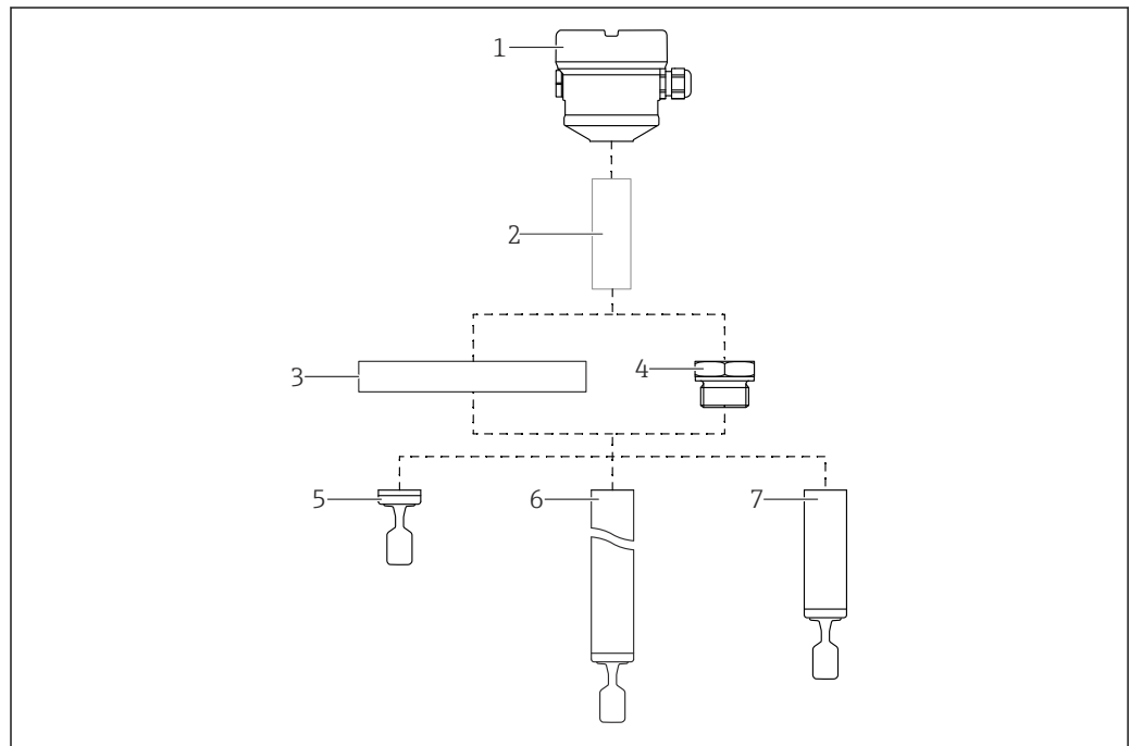
图 2 产品设计: Liquiphant FTL51B
