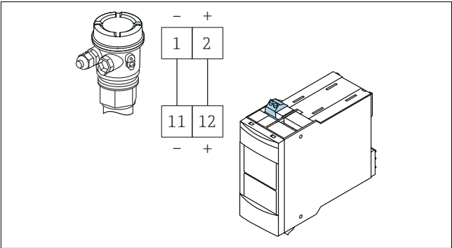
图 2 使用电源线连接传感器
