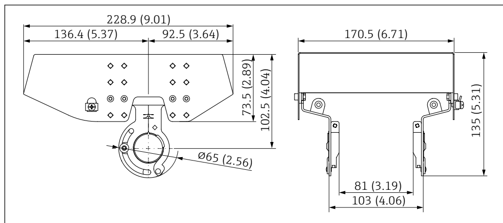
64 Dimensioni del tettuccio di protezione dalle intemperie, 316 L, XW112. Unità di misura mm (in)
