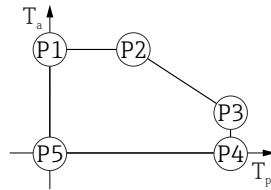
11 Custodia in plastica; temperatura di processo 0 ... +150 °C (+32 ... +302 °F) con approvazione CSA C/US
