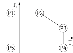
12 Custodia in plastica; temperatura di processo -20 ... +200 °C (-4 ... +392 °F)
