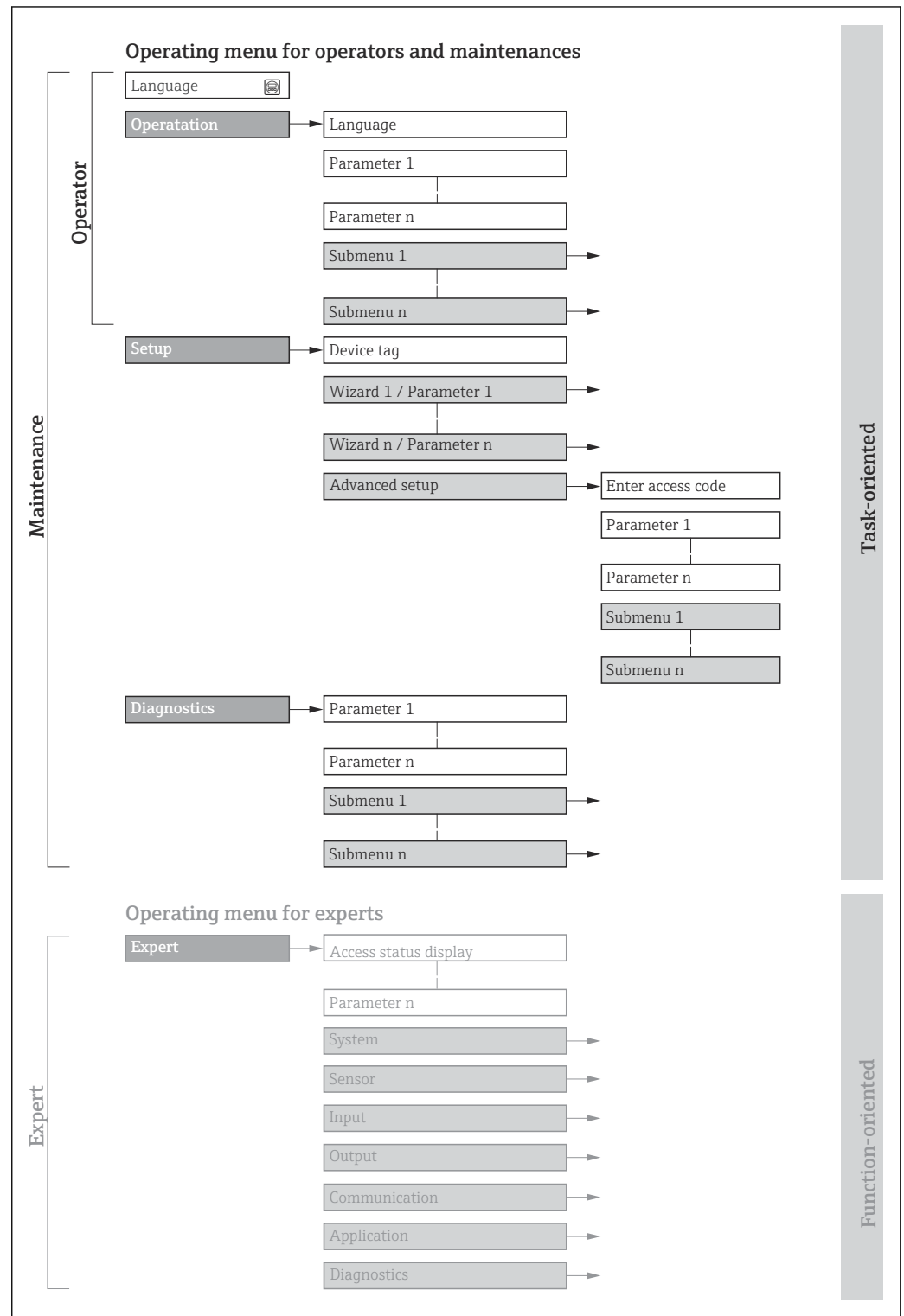
15 Схематичная структура меню управления
