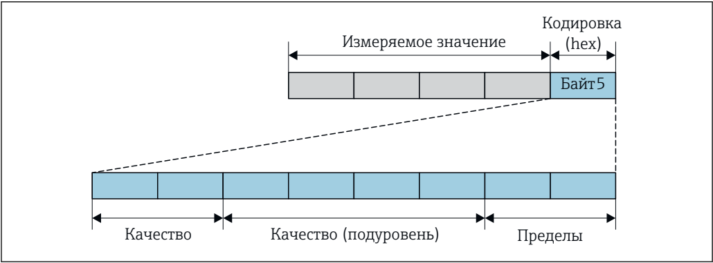
22 Структура байта кодирования
