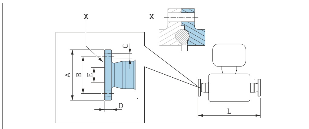
25 Detalhe X: Conexão de processo assimétrica; a peça exibida em cinza é fornecida pelo fornecedor.
