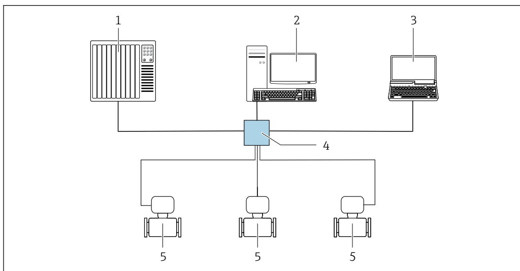
45 Opções para operação remota através da rede EtherNet/IP: topologia estrela
