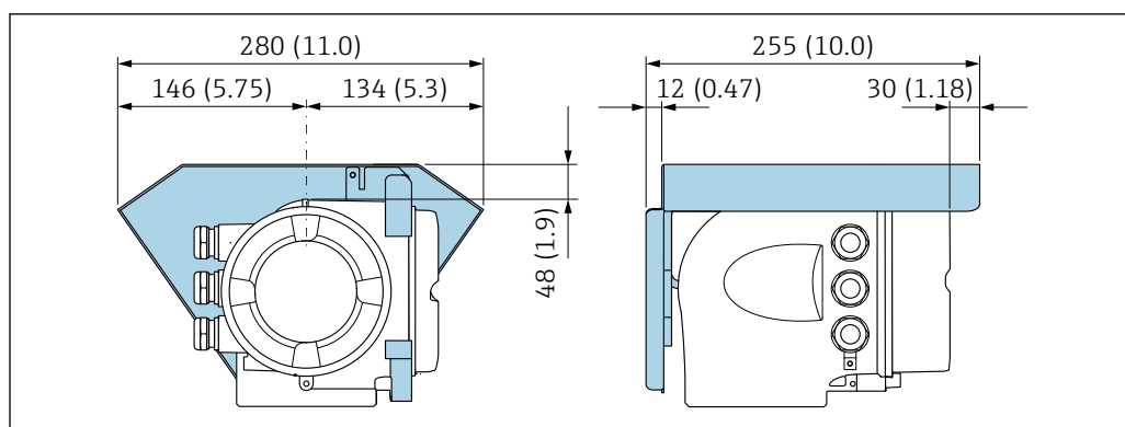
26 Unidade em mm (pol.)
