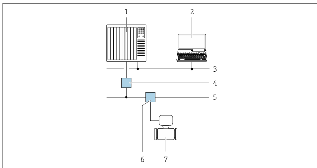
41 Opções para operação remota através da rede PROFIBUS PA
