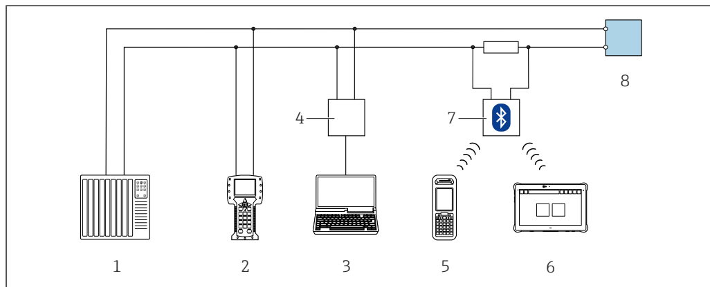
37 Opções para operação remota através do protocolo HART (ativa)
