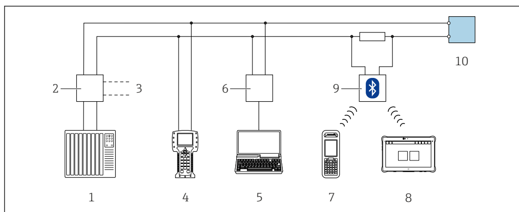
38 Opções para operação remota através do protocolo HART (passiva)
