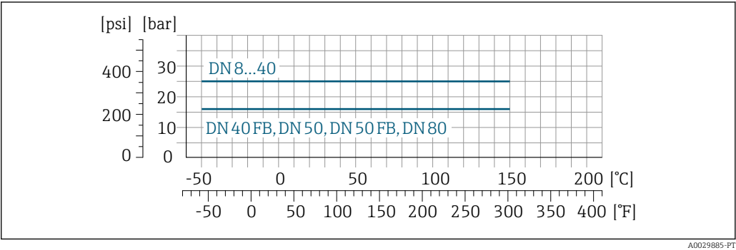
19 Material de flange em titânio Classe 2
