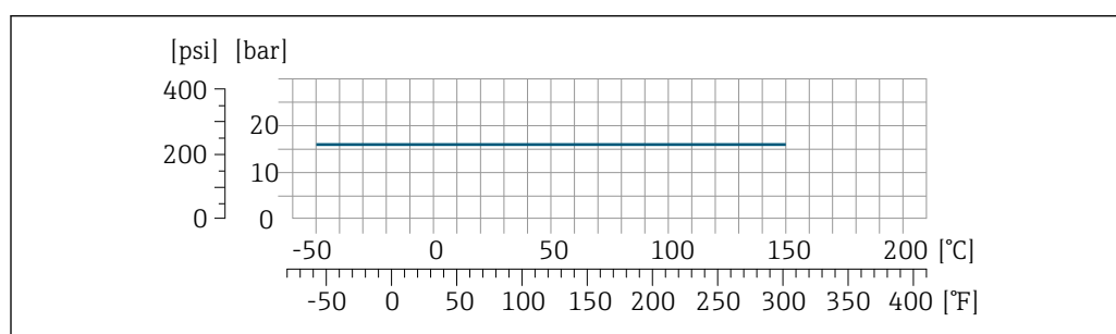
22 Material da conexão em titânio Classe 2
