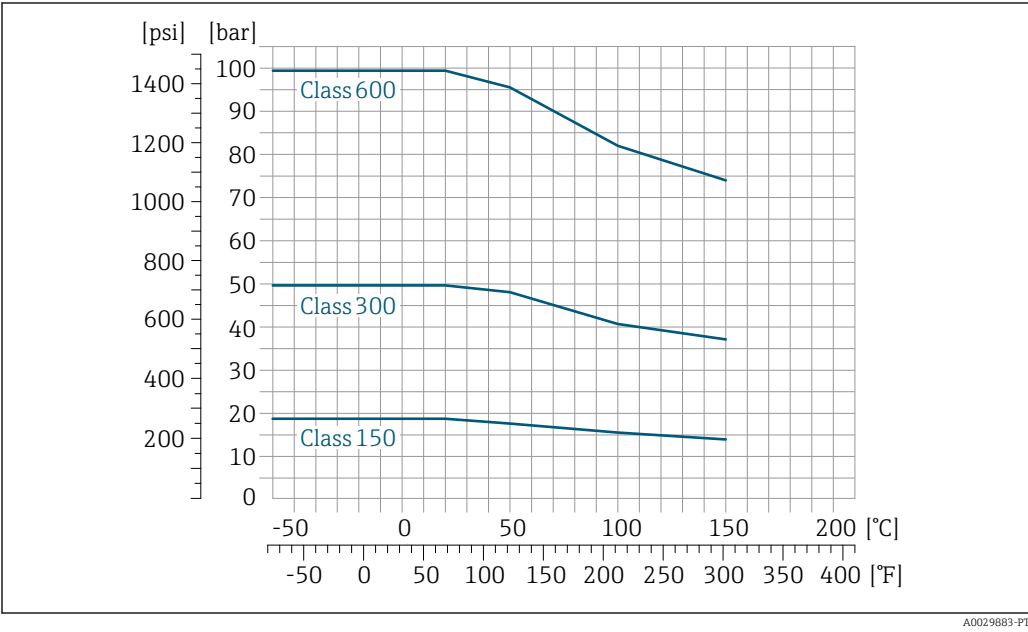
17 Com material de flange 1.4301 (304); peças úmidas: titânio
