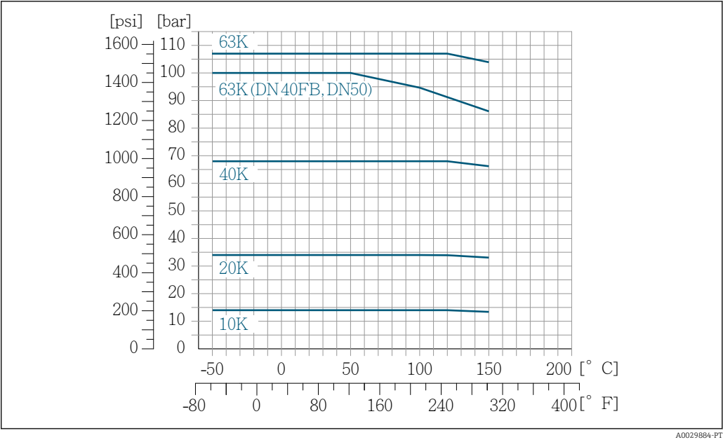
18 Com material de flange 1.4301 (304). Peças úmidas: titânio.
