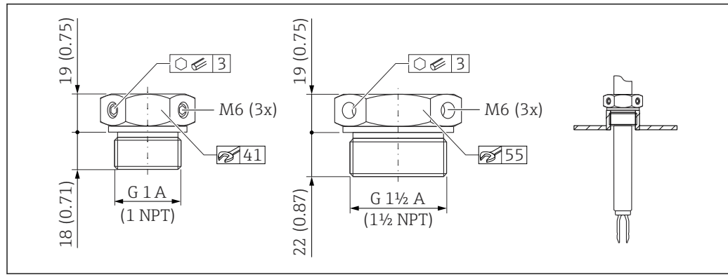
图 49 常压滑动套管 p_e = 0 \text{ bar} (0 psi)。测量单位 mm (in)
