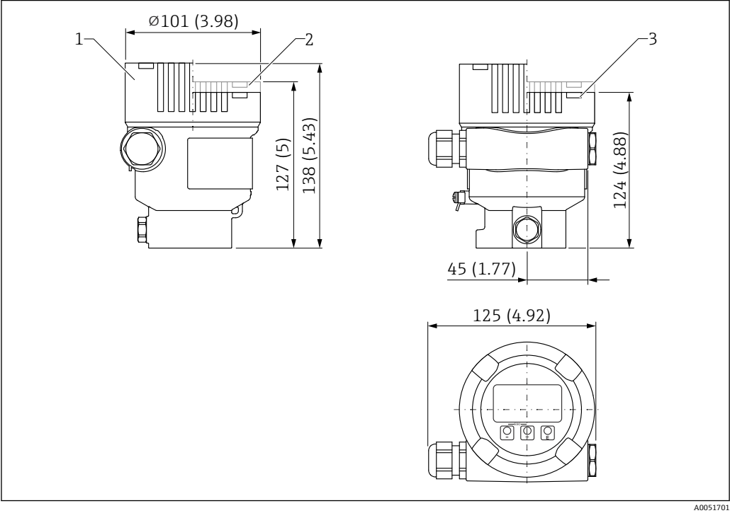
图 24 单腔体铝外壳（带涂层）的外形尺寸示意图。测量单位 mm (in)
