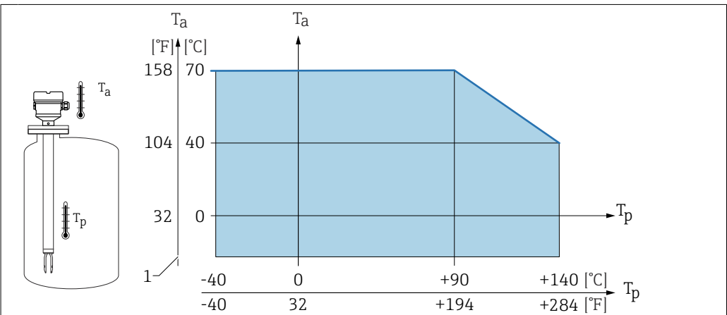
图 19 外壳允许环境温度 T_a 与罐体内部过程温度 T_p 的关系
