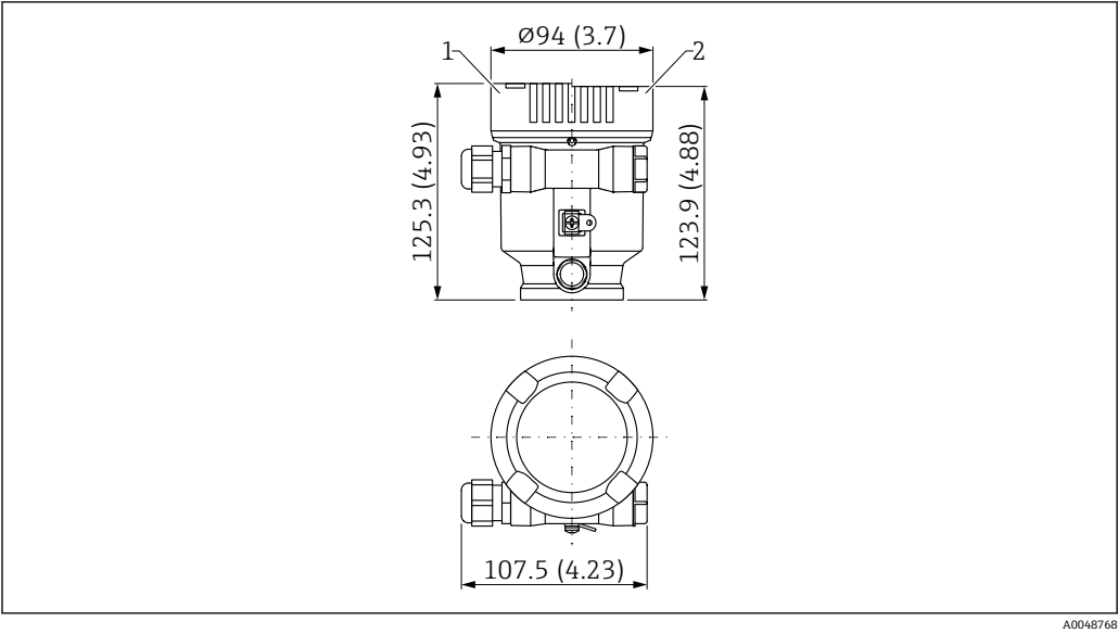
图 23 单腔室塑料外壳的外形尺寸示意图；包括 M20 接头和塑料插头。测量单位 mm (in)
