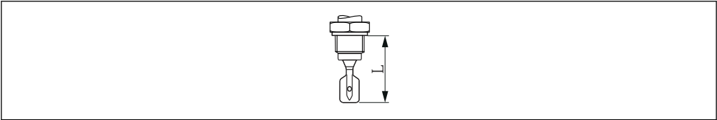
图 29 探头类型：一体式；传感器长度 L
