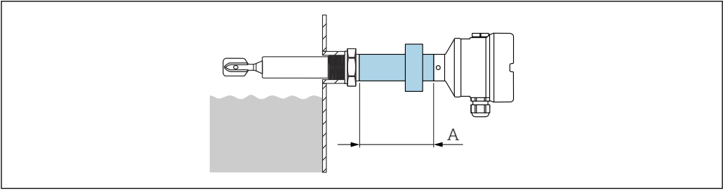
图 28 隔爆玻璃馈通（搭配带延长管的仪表使用）
