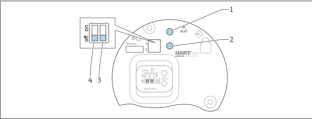
图 44 FEL60H 电子插件上的操作按键和 DIP 开关
