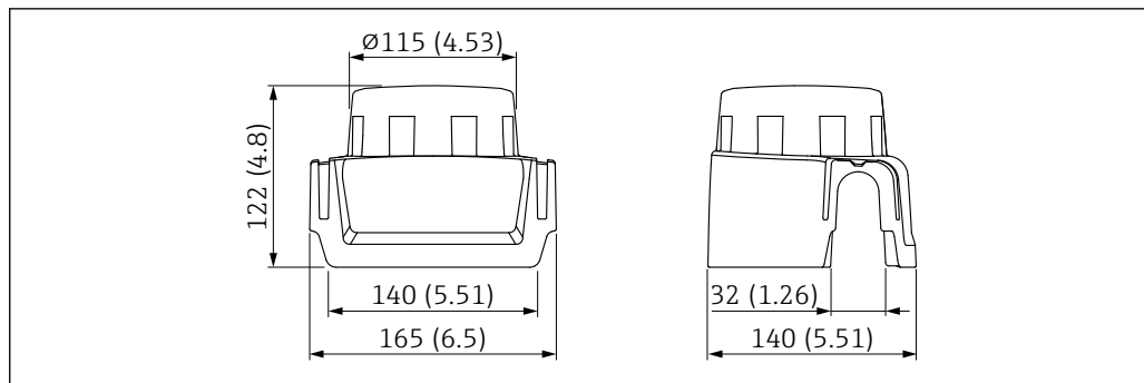
图 47 防护罩，适用单腔体铝外壳。测量单位 mm (in)
