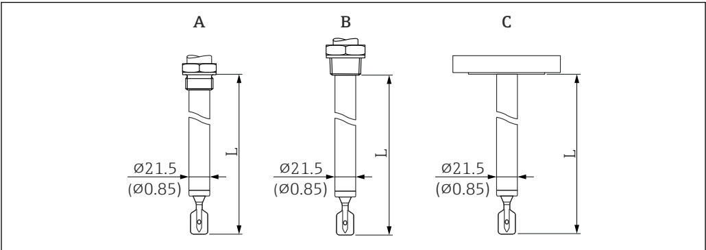
图 30 探头类型：延长管型、短管型（传感器长度 L）。测量单位 mm (in)
