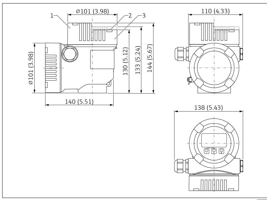
图 26 L 型双腔室铝外壳（带涂层）的外形尺寸示意图；包括 M20 接头和塑料插头。测量单位 mm (in)
