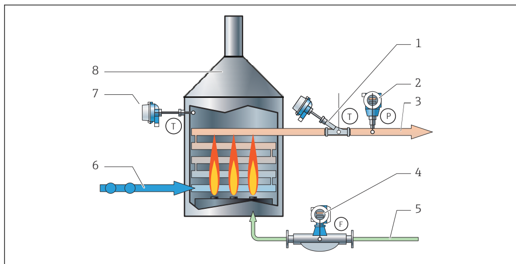
2 Beispiel Messanordnung
