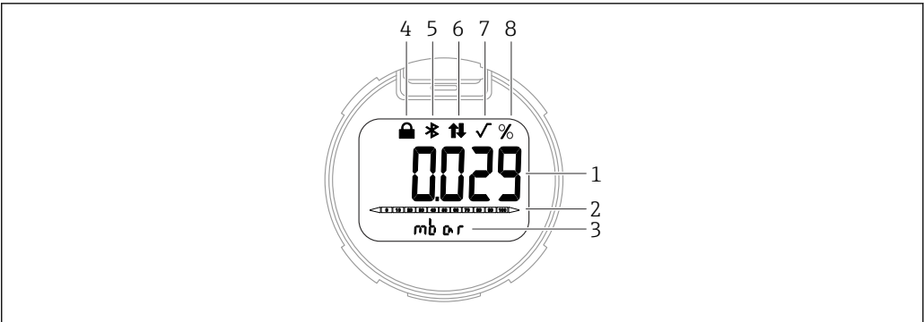
图 10 段码显示屏
