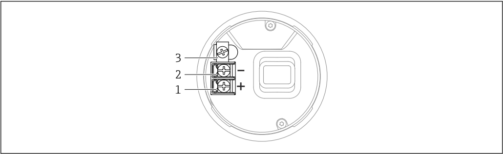
1 接线腔中的接线端子和接地端
