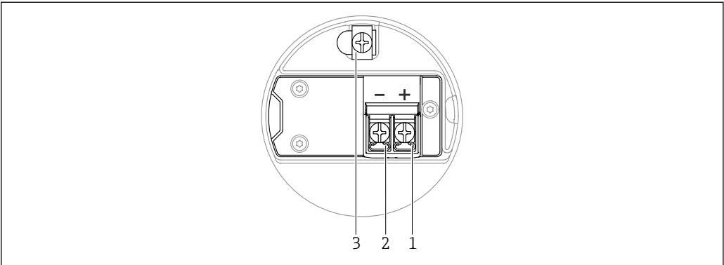
2 接线腔中的接线端子和接地端
