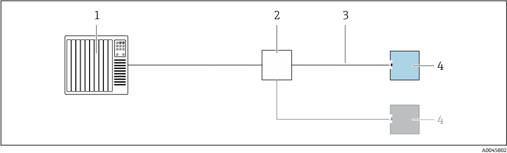
图 5 接线示例：PROFINET + Ethernet-APL
