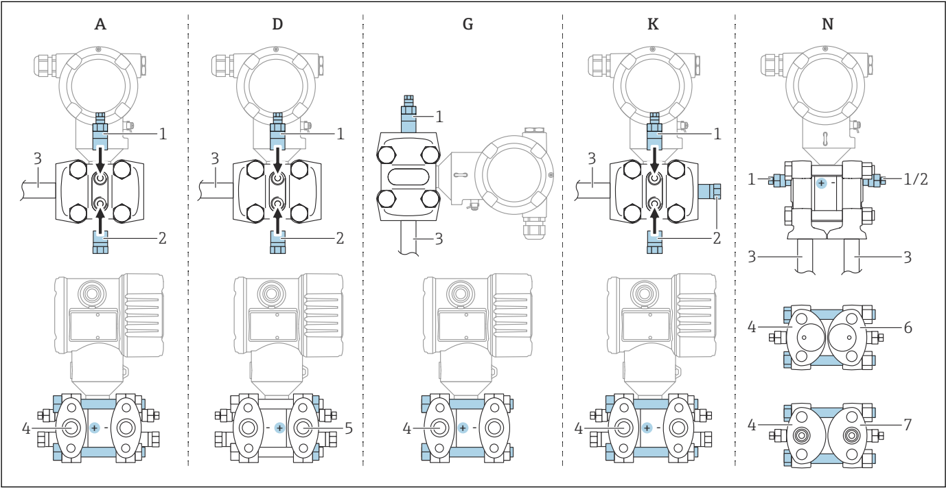
图 6 选型代号: A、D、G、K、N
