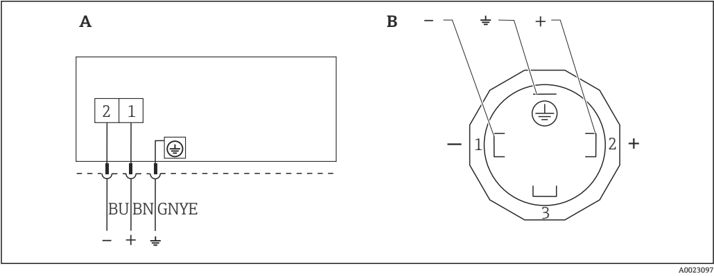
图 3 BN = 棕色，BU = 蓝色，GNYE = 绿/黄相间
