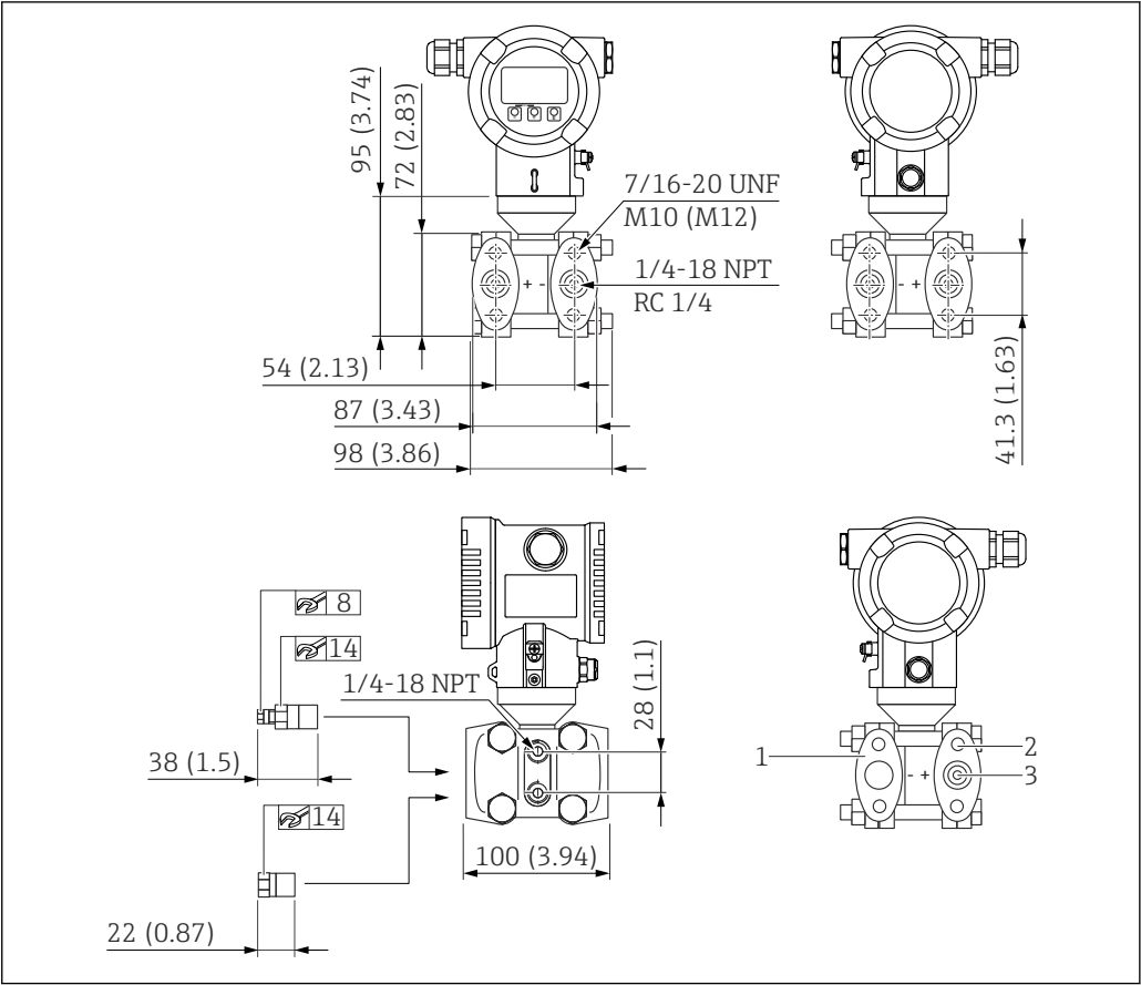
图 9 正视图、左视图、右视图。螺母始终安装在负压侧。测量单位 mm (in)
