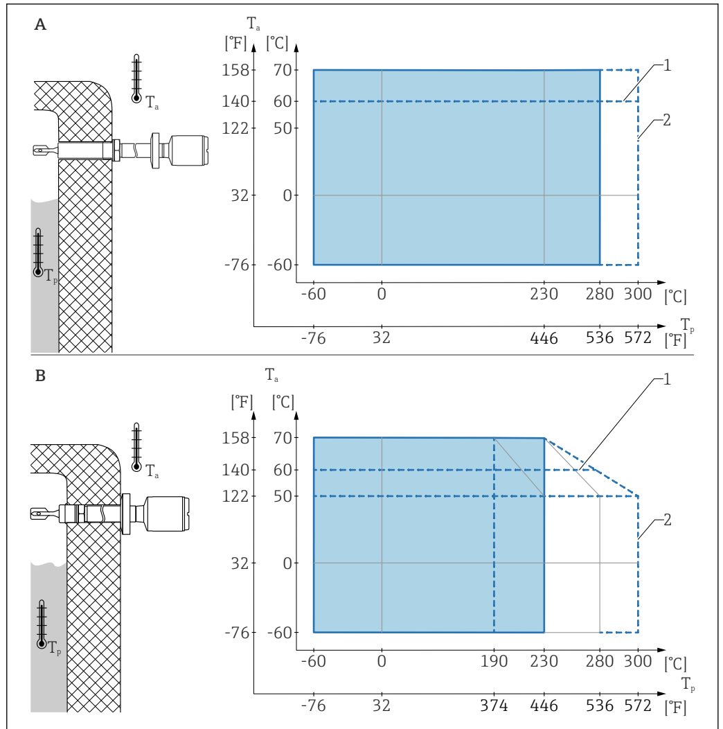
图 49 外壳允许环境温度 T_a 与罐体内部过程温度 T_p 的关系；最高过程温度 230 °C (446 °F) 或 280 °C (536 °F)
