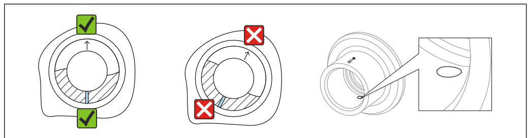
图 11 焊座，带泄漏检测孔
