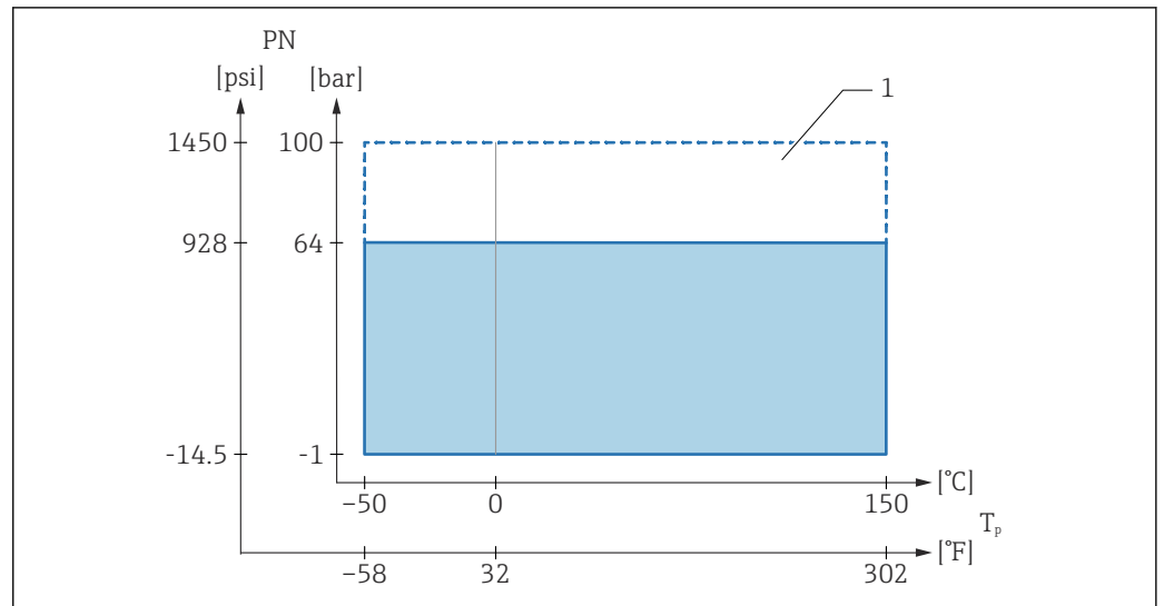
图 50 过程压力范围 (过程温度 T_p 不超过 150 °C (300 °F) 时)
