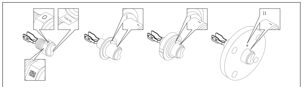
图 12 参照标记水平安装在罐体中的音叉位置
