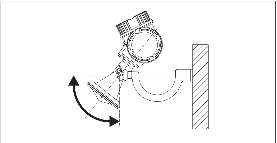
7 Instalação da antena piramidal com suporte de montagem (FMR50/FMR56)
