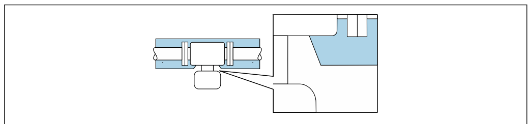
29 Coibentazione con collo esteso a vista
