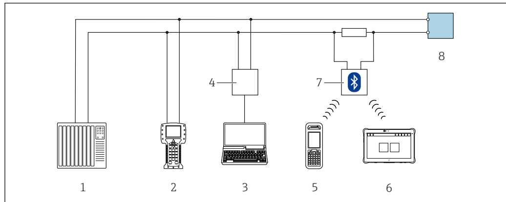
43 Opzioni per funzionamento a distanza mediante protocollo HART (attivo)
