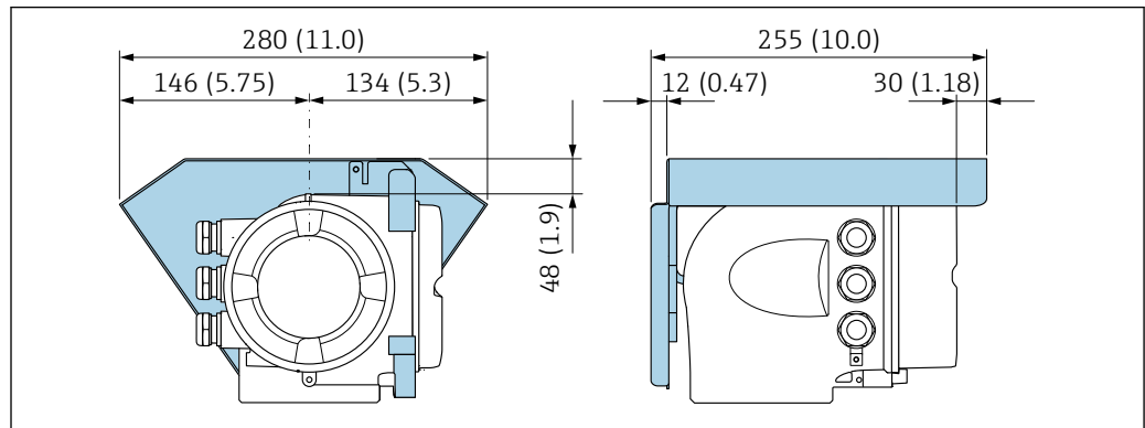
36 Unità mm (in)
