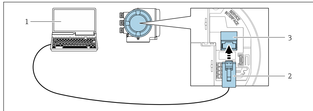
55 Connessione mediante interfaccia service (CDI-RJ45)
