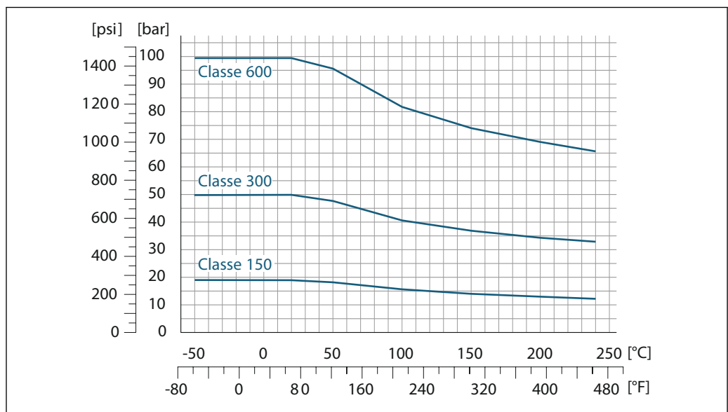
22 Con materiale flangia 1.4301 (F304); parti bagnate Alloy C22
