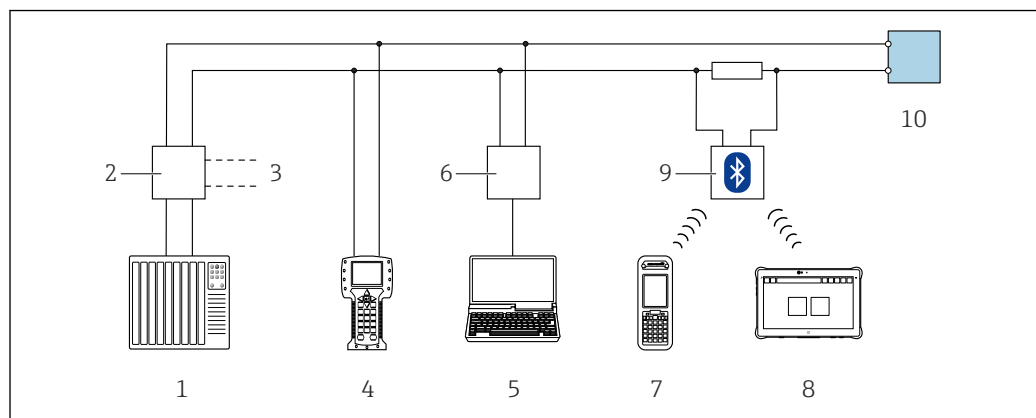
44 Opzioni per funzionamento a distanza mediante protocollo HART (passivo)
