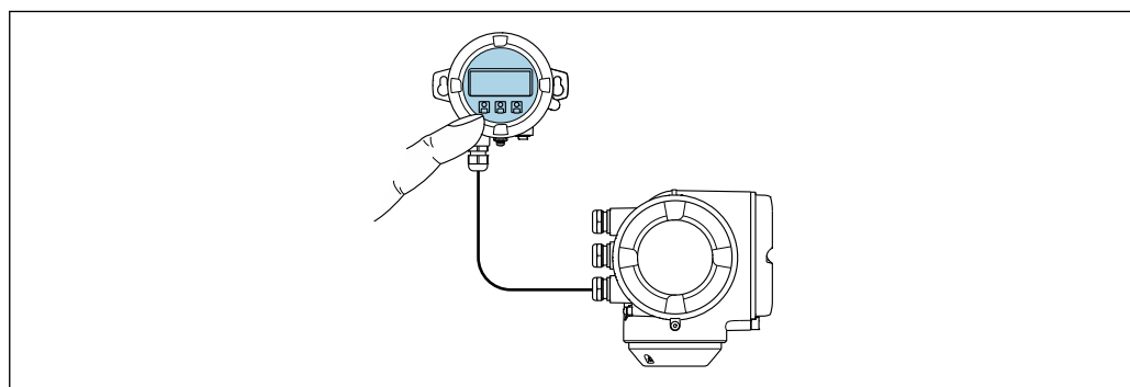
☒ 42 Operatività mediante modulo di visualizzazione e controllo separato DKX001
