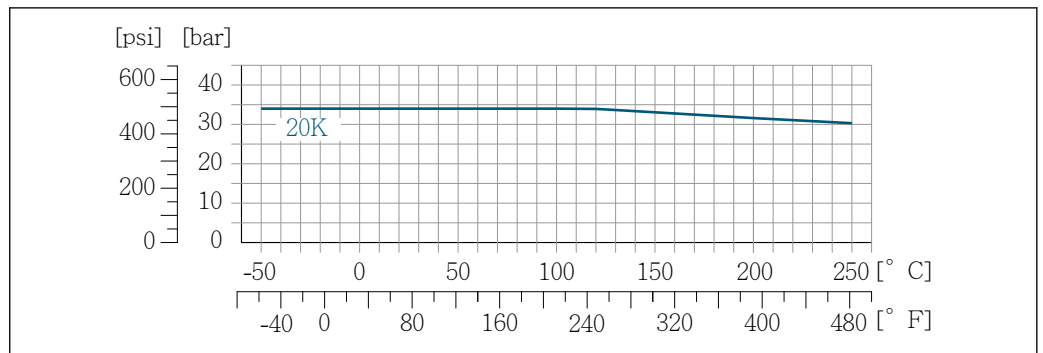
23 Con materiale flangia 1.4301 (F304); parti bagnate Alloy C22
