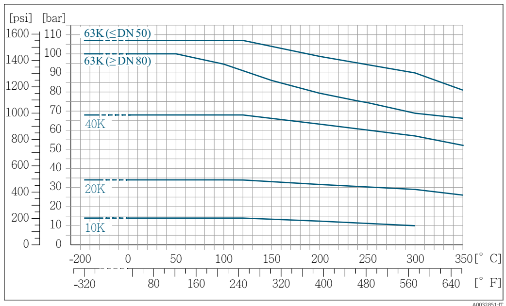
19 Con materiale flangia 1.4404 (F316/F316L), Alloy C22
