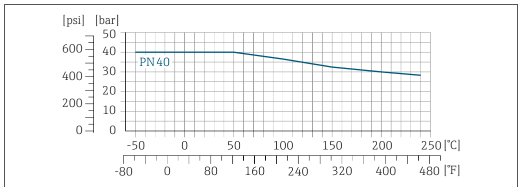
21 Con materiale flangia 1.4301 (F304); parti bagnate Alloy C22
