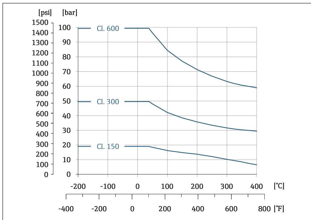
图 18 连接法兰的材质：不锈钢 1.4404/F316/F316L，多种材料认证
