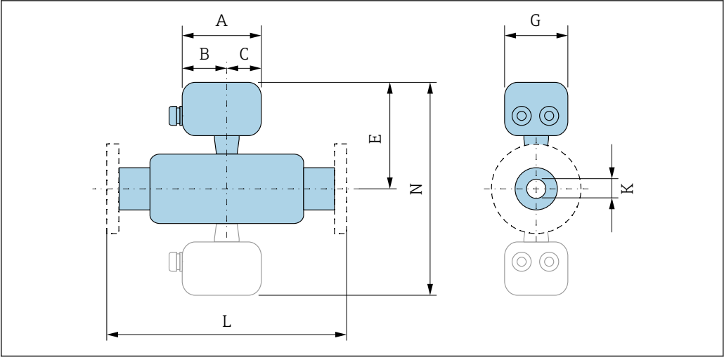
24 灰色区域: 双传感器型
