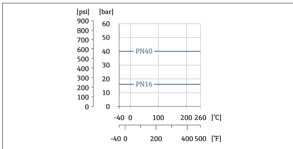
图 17 连接法兰的材质：铸造合金 2.4602/UNS N06022，类似 Alloy C22/2.4602 合金
