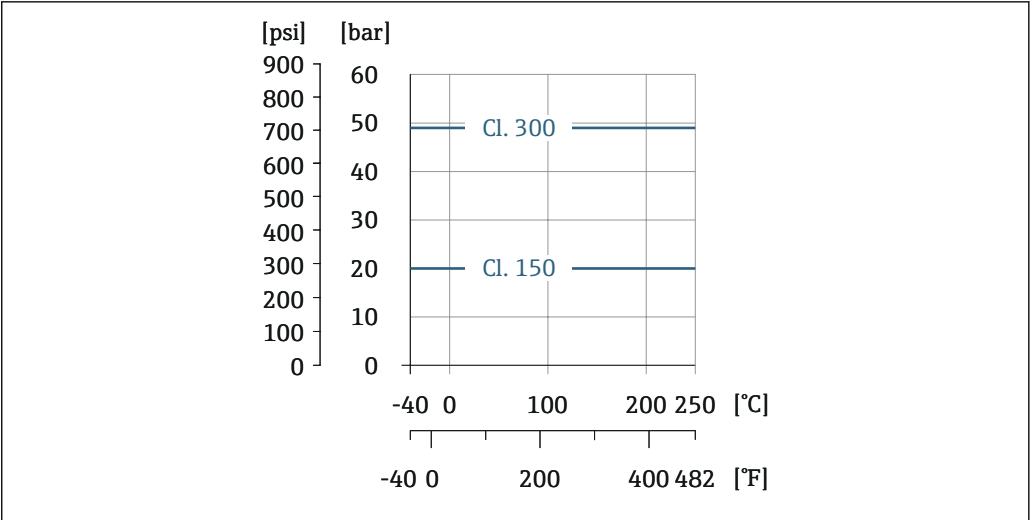
19 连接法兰的材质: 铸造合金 CX2MW, 类似 Alloy C22/2.4602 合金
