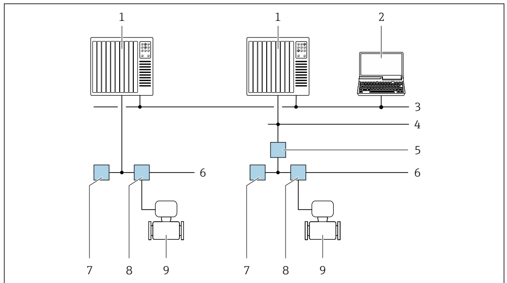
图 31 通过 FOUNDATION Fieldbus 网络进行远程操作
