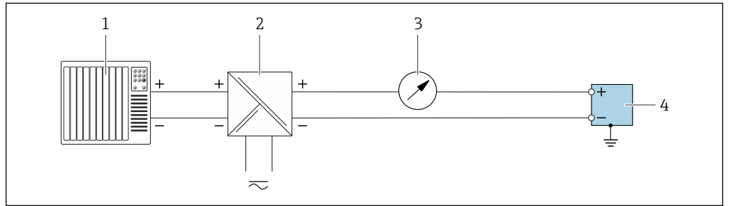
图 6 接线实例：4 ... 20 mA 电流输出 (无源)
