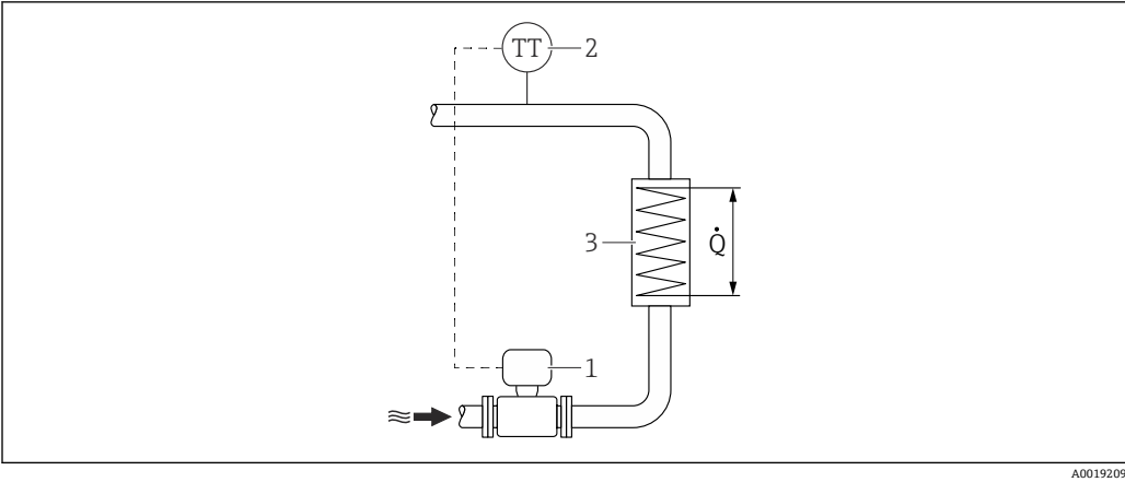
15 蒸汽和水热量差值测量示意图
