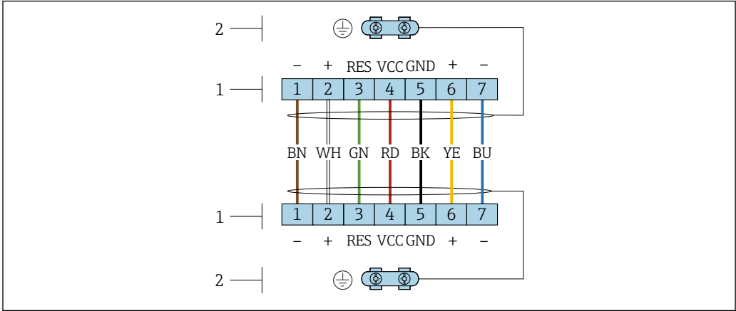
图 4 变送器墙装架中的接线腔和传感器接线盒内的接线端子
