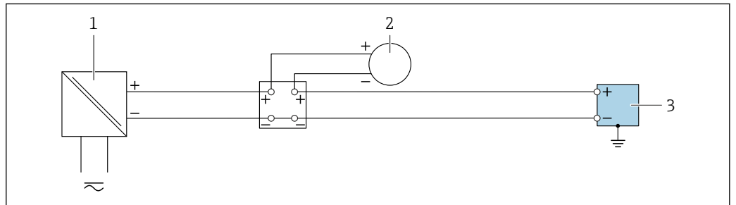
图 7 接线实例：4 ... 20 mA 电流输入
