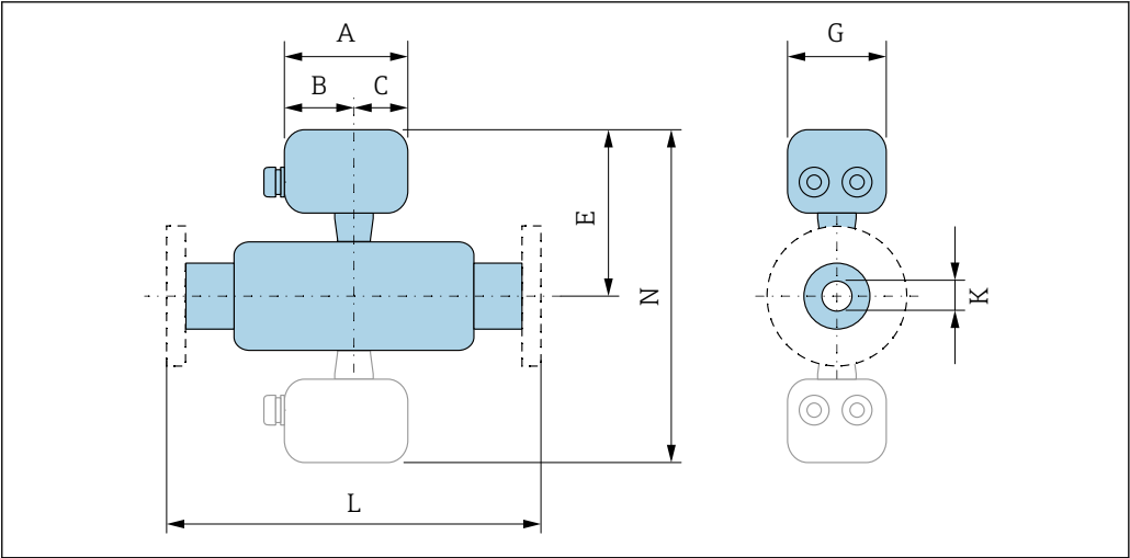
26 灰色区域：双传感器型
