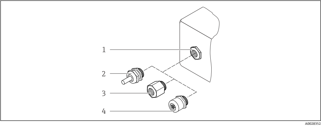
图 27 允许的电缆入口/缆塞
