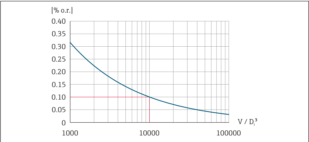
图 11 重复性 = 0.1 % o.r., 体积流量测量值[m³] of V = 10\,000 \cdot D_i^3
