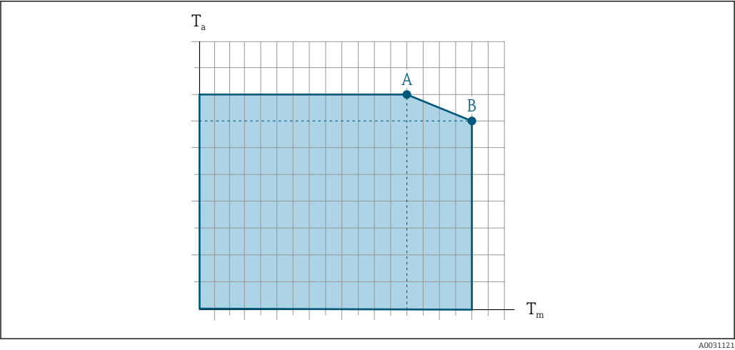
36 Beispielhafte Darstellung, Werte in der nachfolgenden Tabelle. T_a Umgebungstemperatur T_m Messstofftemperatur A Maximal zulässige Messstofftemperatur T_m bei T_{a\,max} = 60\text{ °C (140 °F)} ; höhere Messstofftemperaturen T_m erfordern eine Reduktion der Umgebungstemperatur T_a B Maximal zulässige Umgebungstemperatur T_a bei der maximal spezifizierten Messstofftemperatur T_m des Messaufnehmers
