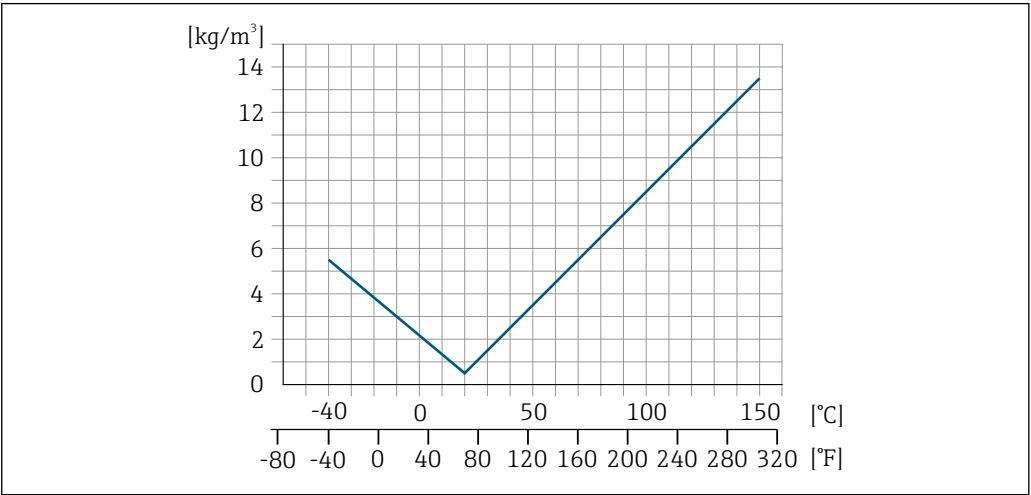
42 Ajustage sur site de la masse volumique, par exemple à +20 °C (+68 °F)
