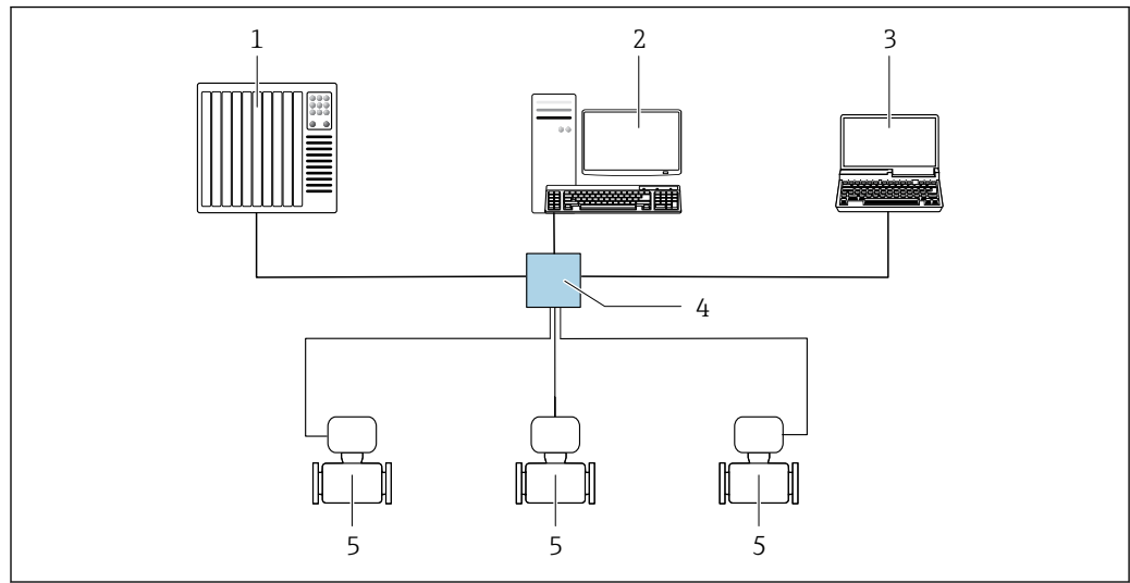
31 Options pour la configuration à distance via le réseau EtherNet/IP : topologie en étoile
