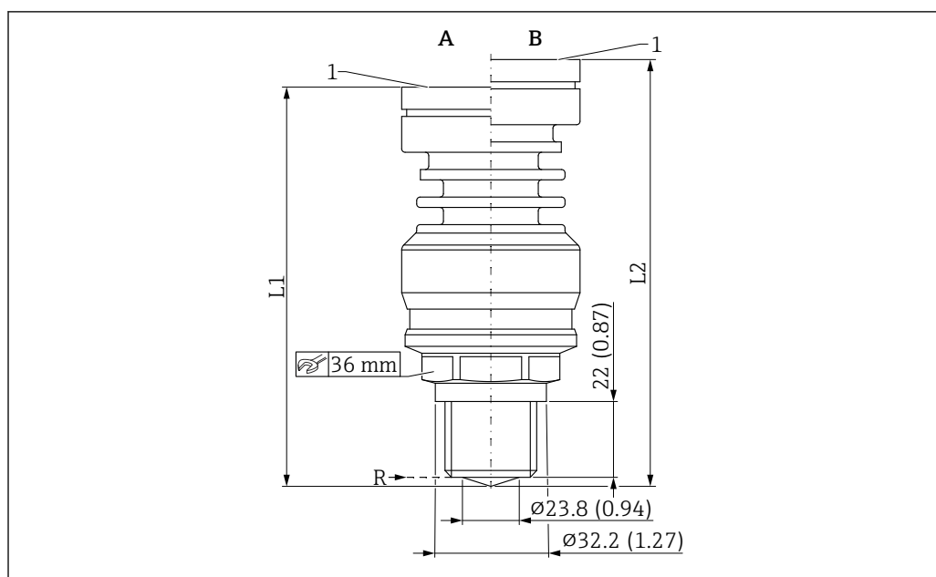
56 Medidas; antena integrada, PEEK, 20 mm (0,75 in); conexión a proceso, rosca de ¾". Unidad de medida mm (in)
