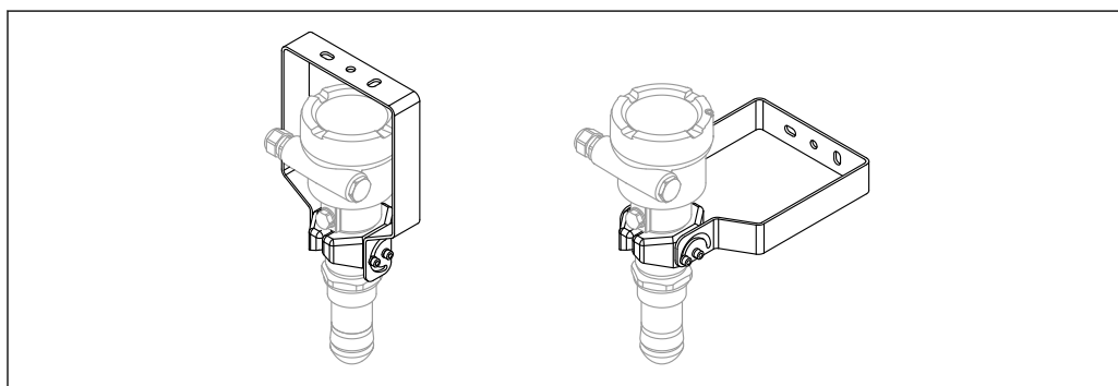
66 Soporte de montaje ajustable FMR6xB; montaje en pared o en techo
