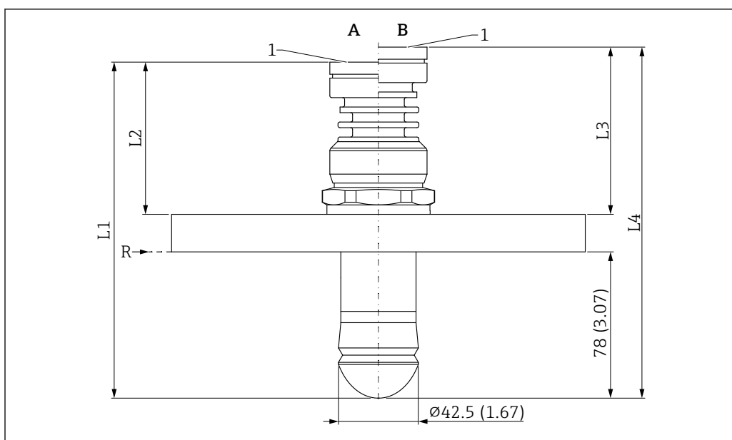
■ 52 Medidas de la antena de goteo 50 mm (2 in), conexión a proceso: brida UNI. Unidad de medida mm (in)
