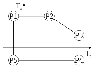
14 Caja de plástico; temperatura de proceso -40 \dots +80 \text{ }^{\circ}\text{C} ( -40 \dots +176 \text{ }^{\circ}\text{F} )
