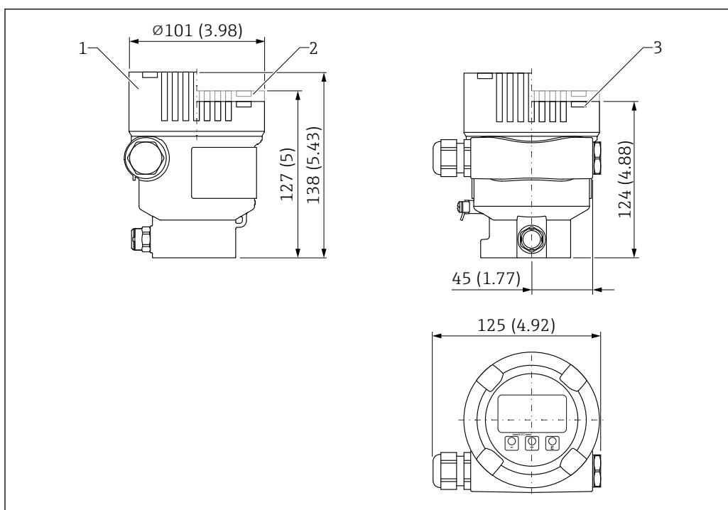
41 Medidas; caja de compartimento único, aluminio, recubierto; incl. acoplamiento M20 y tapón, plástico. Unidad de medida mm (in)
