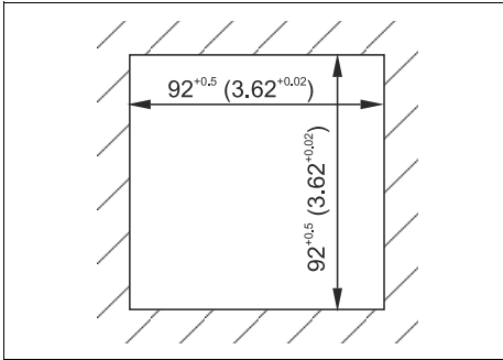
Abb. 1: Schaltschrankschnitt in mm (inch)
