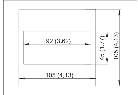
Abb. 2: Adapterrahmen im eingebauten Zustand
