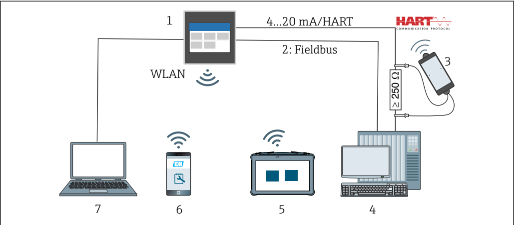
图 30 系统集成
