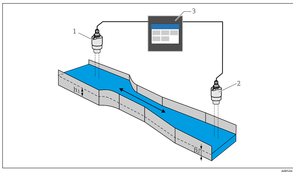
图 36 回水检测
