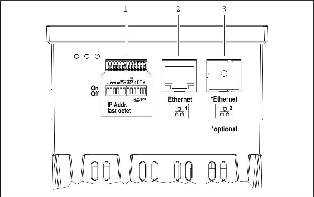
19 盘装型设备的连接口（设备底部）
