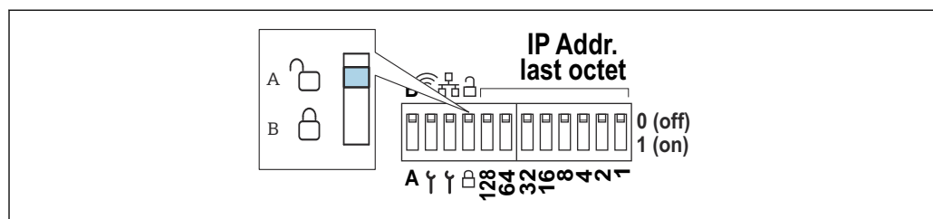
39 通过 DIP 开关进行硬件锁定
