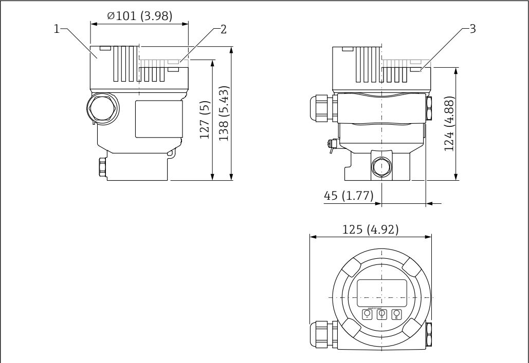
图 27 单腔体铝外壳（带涂层）的外形尺寸示意图。测量单位 mm (in)
