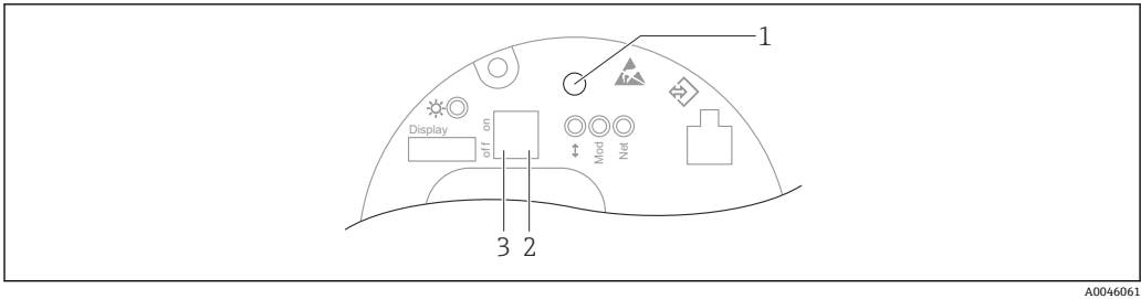
图 48 Ethernet-APL 通信型电子插件 (FEL60P) 上的操作按键和 DIP 开关
