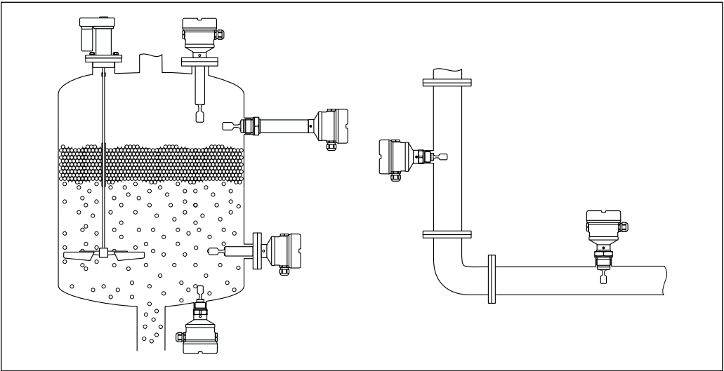
10 安装实例：安装在容器、罐体或管道中
