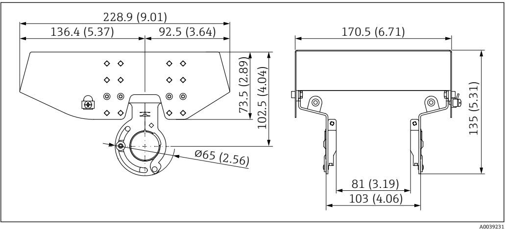
图 52 316L 防护罩 XW112 的外形尺寸示意图。测量单位 mm (in)
