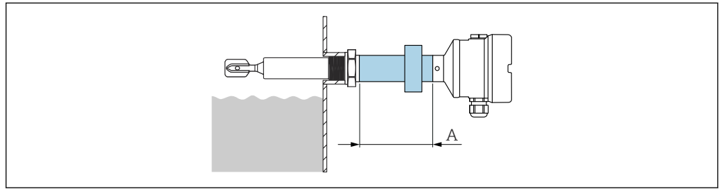
图 31 隔爆玻璃馈通（搭配延长管使用）
