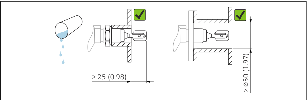
11 安装实例：测量低粘度液体。测量单位 mm (in)
