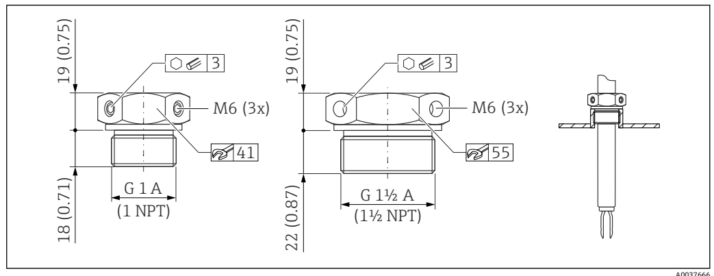
55 常压滑动套管 p_e = 0 bar (0 psi)。测量单位 mm (in)
