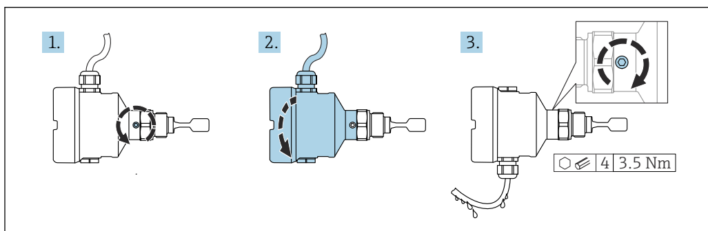
图 18 外壳带固定螺丝；在电缆上建立排水回路
