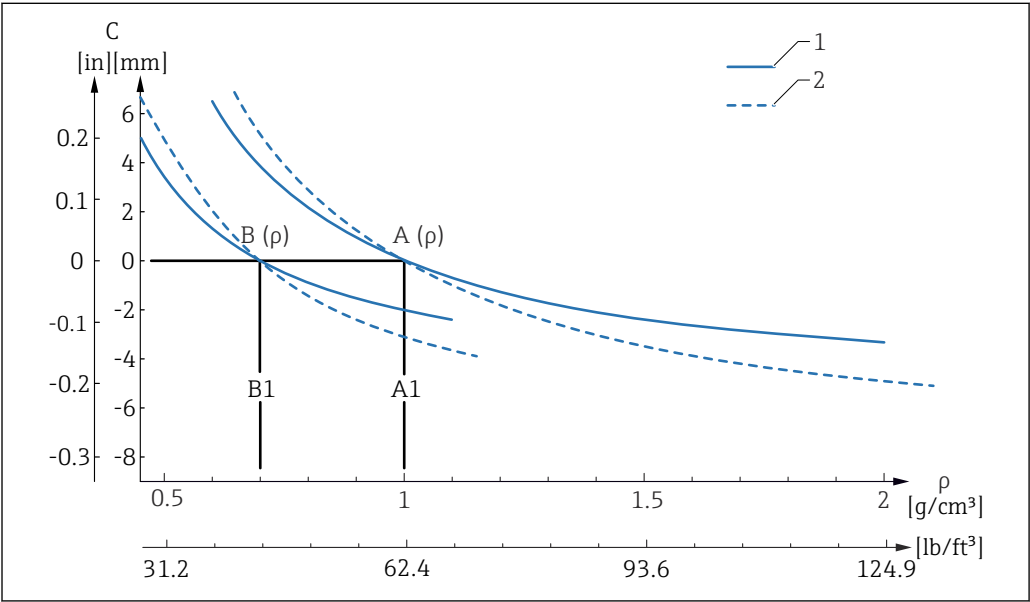
图 9 参考开关点偏差随密度的变化而变化 A 密度设定值 ( \rho ) > 0.7 \text{ g/cm}^3 (43.7 lb/ft 3 ) A1 参考条件 \rho = 1 \text{ g/cm}^3 (62.4 lb/ft 3 ) B 密度设定值 ( \rho ) > 0.5 \text{ g/cm}^3 (31.21 lb/ft 3 ) B1 参考条件 \rho = 0.7 \text{ g/cm}^3 (43.7 lb/ft 3 ) C 开关点偏差 1 材质: 316L 2 材质: Alloy C22 合金
