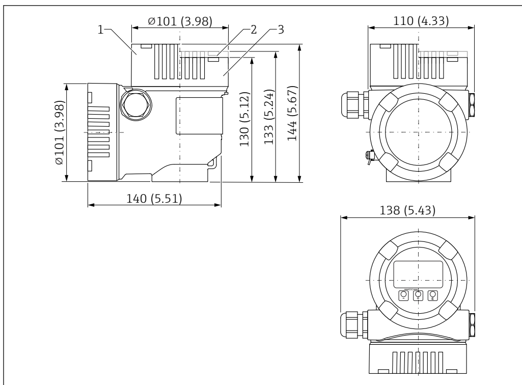
图 30 L 型双腔室 316L 外壳的外形尺寸示意图；包括 M20 接头和塑料插头。测量单位 mm (in)
