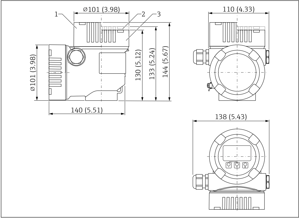
图 29 L 型双腔室铝外壳（带涂层）的外形尺寸示意图；包括 M20 接头和塑料插头。测量单位 mm (in) 1 带玻璃观察窗的盖板高度（适用 Ex d/XP 和粉尘防爆仪表） 2 带塑料观察窗的盖板高度 3 不带观察窗的盖板高度
