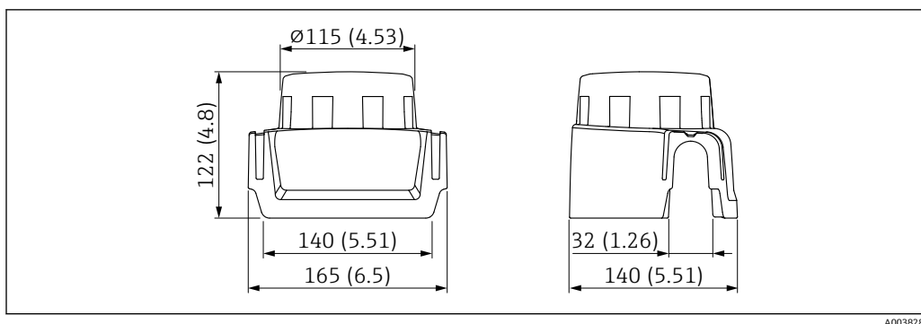
图 53 塑料防护罩 XW111 的外形尺寸示意图。测量单位 mm (in)
