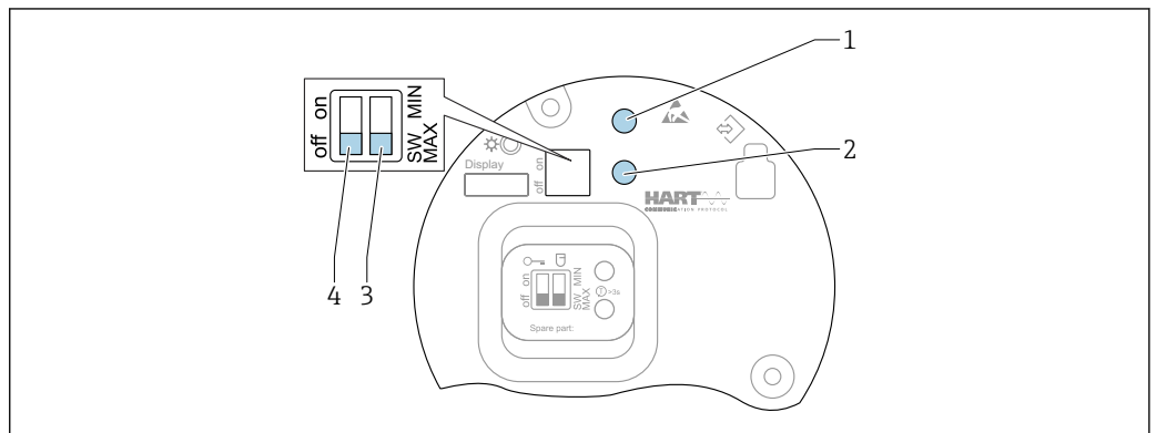
图 47 FEL60H 电子插件上的操作按键和 DIP 开关
