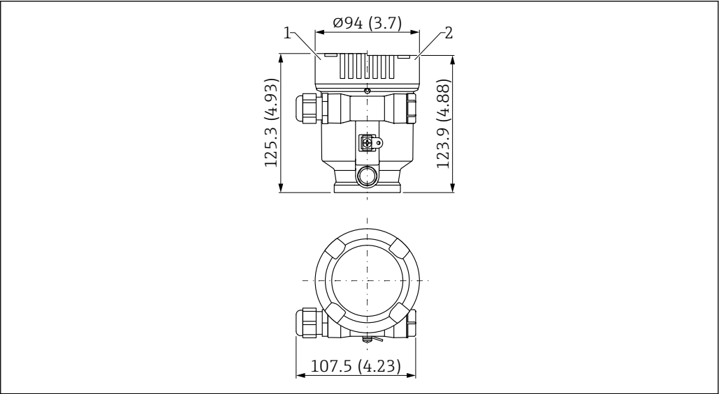
图 26 单腔室塑料外壳的外形尺寸示意图；包括 M20 接头和塑料插头。测量单位 mm (in)
