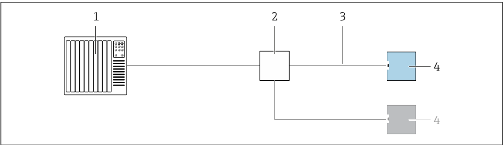
图 6 接线示例：PROFINET + Ethernet-APL
