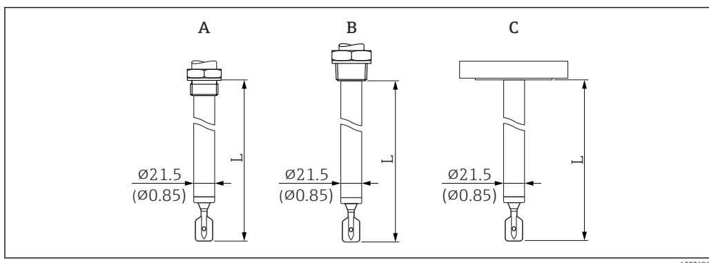
图 33 探头类型：延长管型、短管型（传感器长度 L）。测量单位 mm (in)
