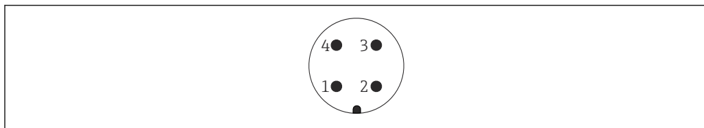
图 4 设备接线示意图
