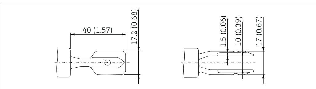
图 34 叉体。测量单位 mm (in)
