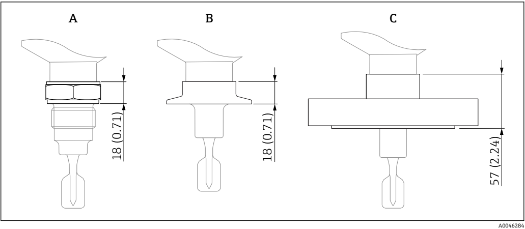
35 过程连接的最大高度规格。测量单位 mm (in)
