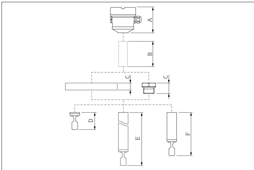
图 25 计算仪表高度所需考虑的部件
