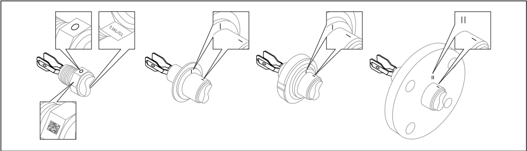
15 参照标记水平安装在罐体中时的音叉位置
