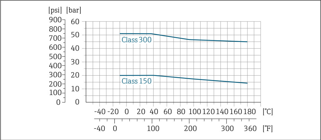
28 Material das conexões de processo: aço carbono, A105
