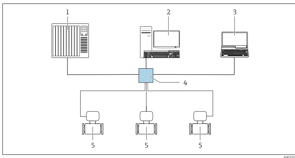
53 Opções para operação remota através da rede EtherNet/IP: topologia estrela
