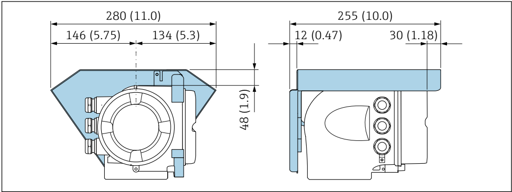
40 Tampa de proteção para Proline 500; unidade mm (pol.)
