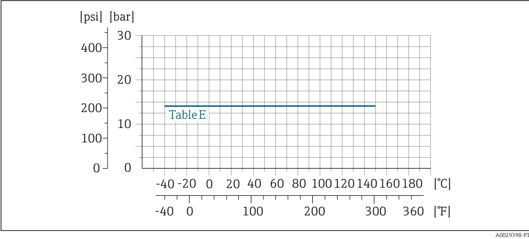
31 Material das conexões de processo: aço carbono, A105/S235JRG2/S275JR
