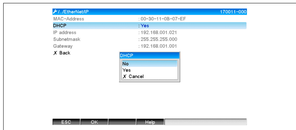
5 Configurações de rede: DHCP desabilitado (operação local)
