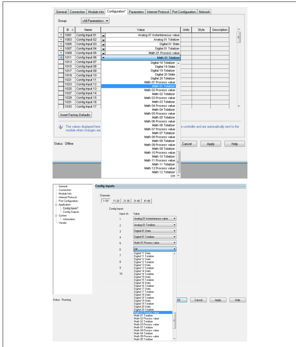
18 Configuração dos dados de entrada/saída usando o Conjunto de Configuração (EDS AOP / AOP Customizado)
