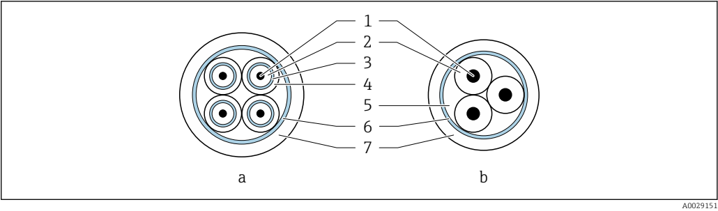
9 Section de câble
