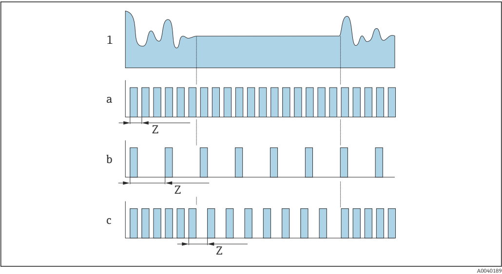
5 Principe de fonctionnement des différentes méthodes d'enregistrement des données
