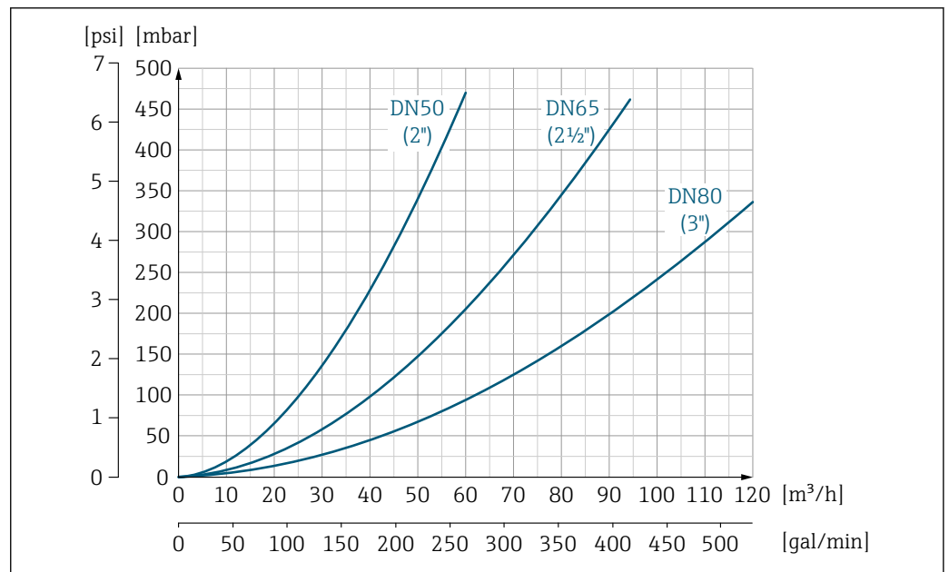
24 Perte de charge DN 50 à 80 (2 to 3") pour caractéristique de commande "Construction", option C "Bride fixe, tube de mesure rétréci", sections d'entrée/de sortie 0 x DN"
