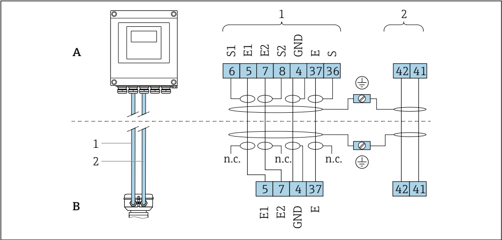
4 Affectation des bornes version séparée
