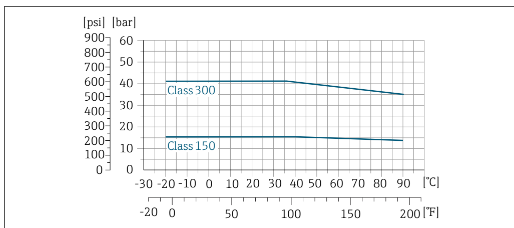
17 Matériau du raccord process : inox
