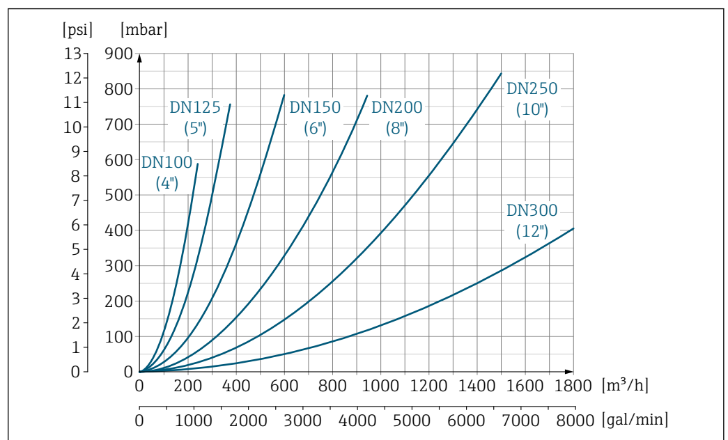
25 Perte de charge DN 100 à 300 (4 to 12") pour caractéristique de commande "Construction", option C "Bride fixe, tube de mesure rétréci", sections d'entrée/de sortie 0 x DN"
