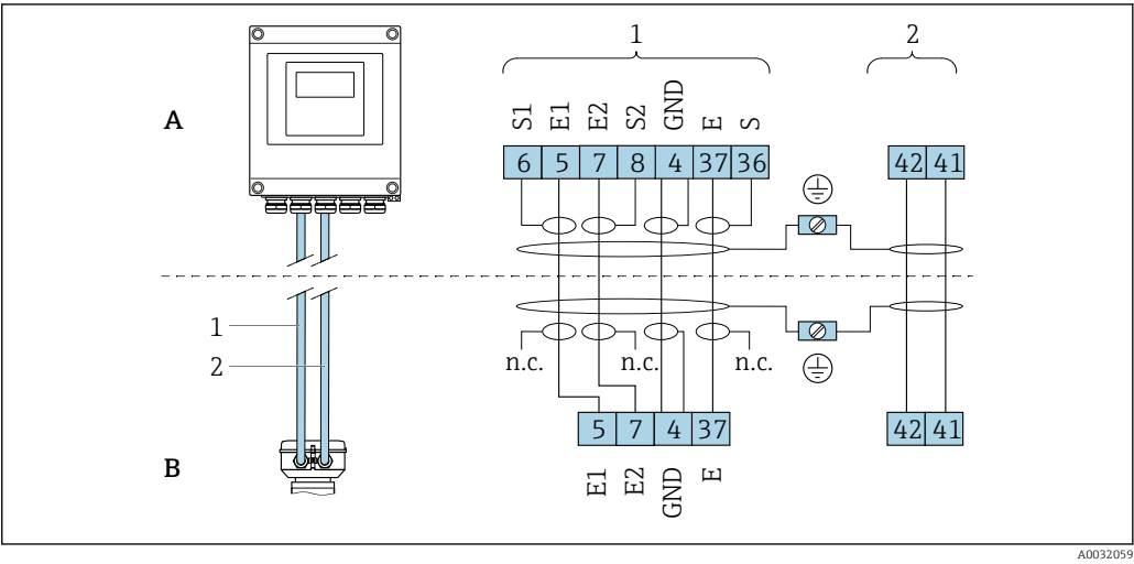
6 Affectation des bornes version séparée
