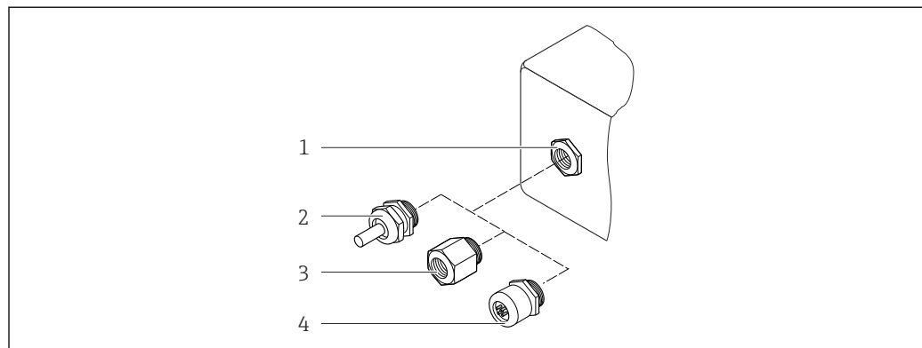
24 Mögliche Kabeleinführungen/-verschraubungen
