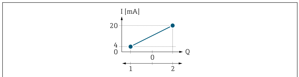
図 4 測定範囲
