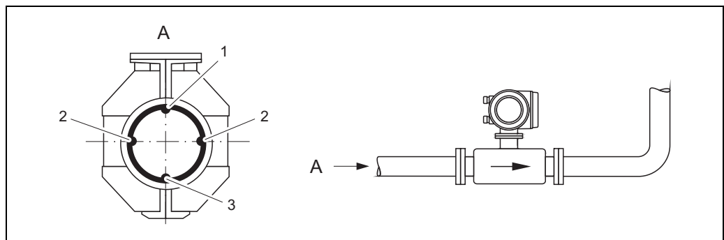
Horizontale Einbaulage
