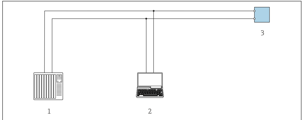
图 23 通过 Modbus RS485 通信进行远程操作（有源信号）
