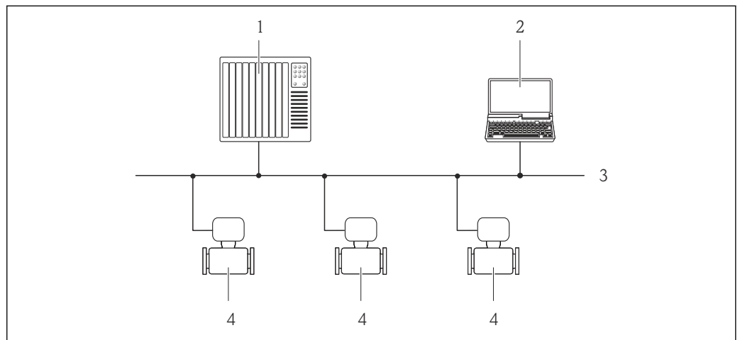
28 Possibilités de configuration à distance via réseau PROFIBUS DP
