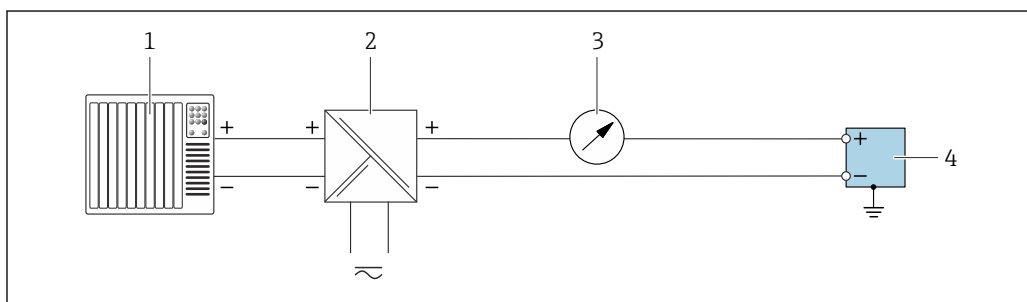
17 Exemple de raccordement pour sortie courant 4 ... 20 mA (passive)
