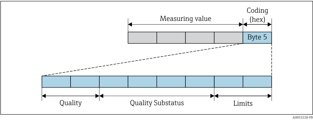
36 Structure de l'octet de codage
