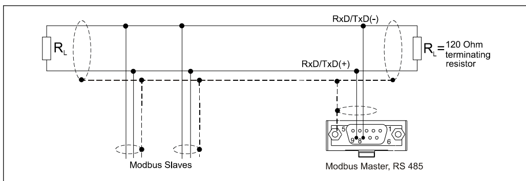
Przyporządkowanie styków złącza Modbus RTU
