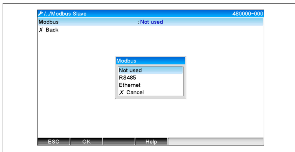
2 Wybór interfejsu komunikacyjnego Modbus
