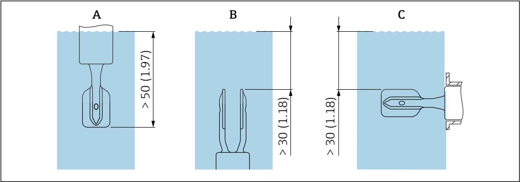
5 单位: mm (in)
