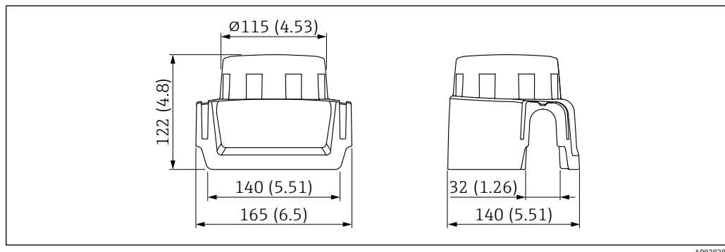
图 23 防护罩，适用单腔体铝外壳。测量单位 mm (in)
