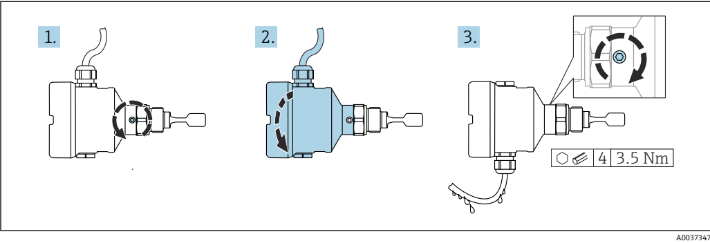
图 17 外壳带外部锁紧螺丝和排水回路
