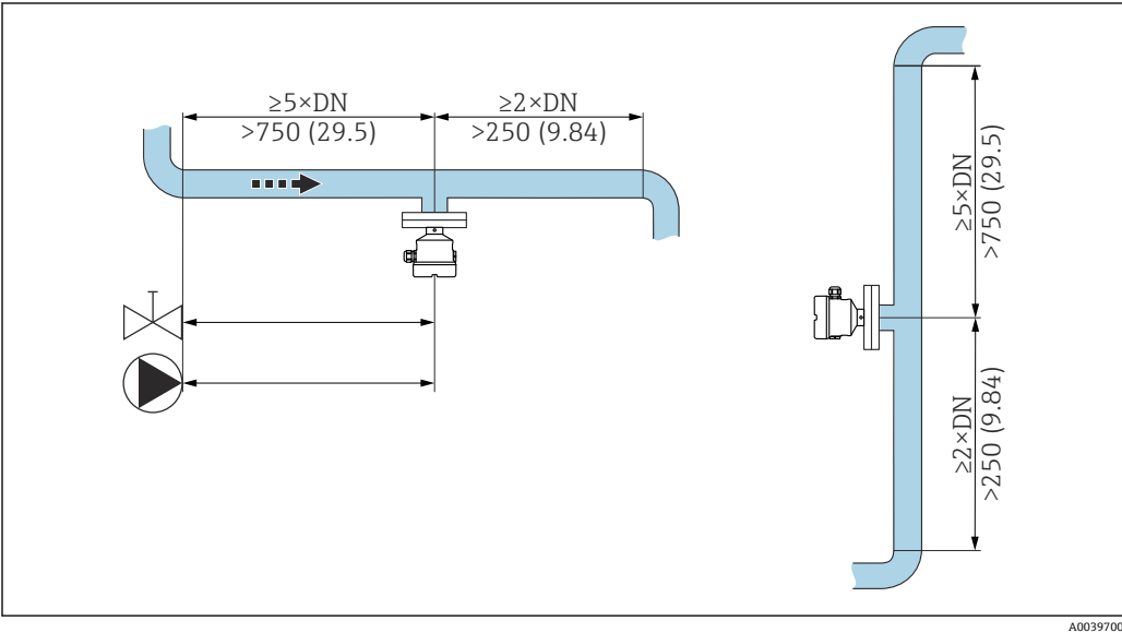
图 8 前直管段的安装。测量单位 mm (in)
