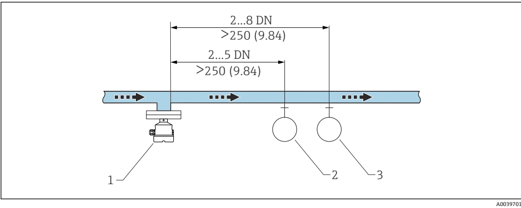
图 9 后直管段的安装。测量单位 mm (in)
