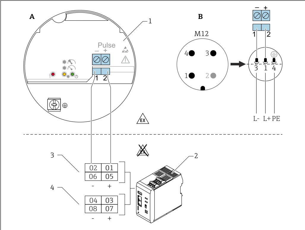
图 19 电子插件 FEL60D 和密度计算仪 QML51 的接线图
