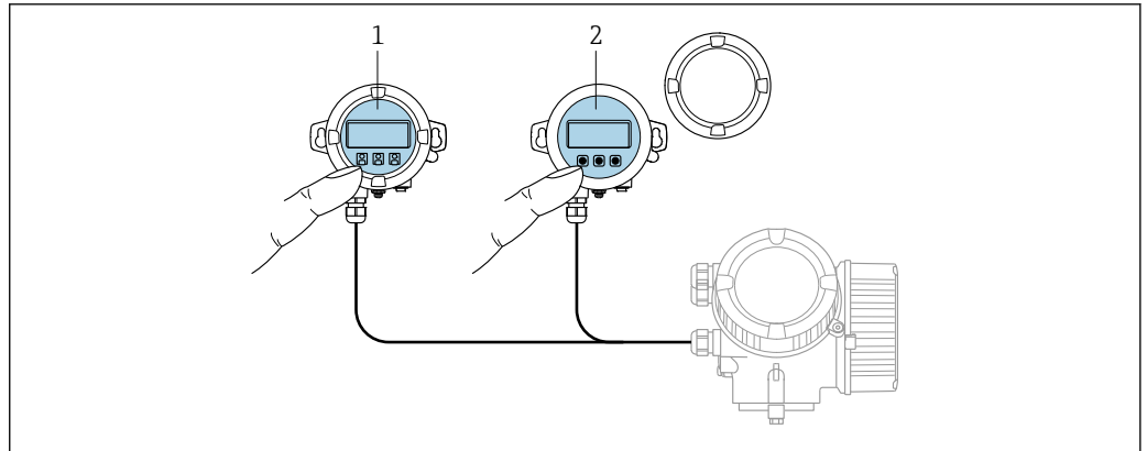
28 Opzioni operative FHX50
