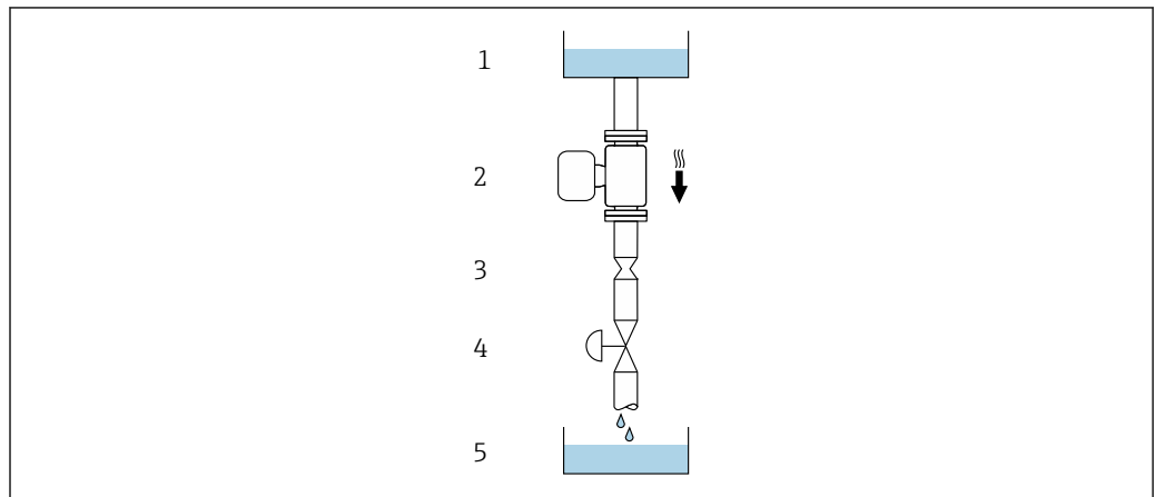
図5 下向き配管への設置 (例：バッチアプリケーション用)
