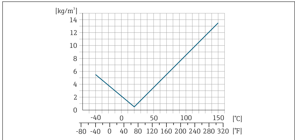
図 34 現場密度調整、例：+20 °C (+68 °F) 時
