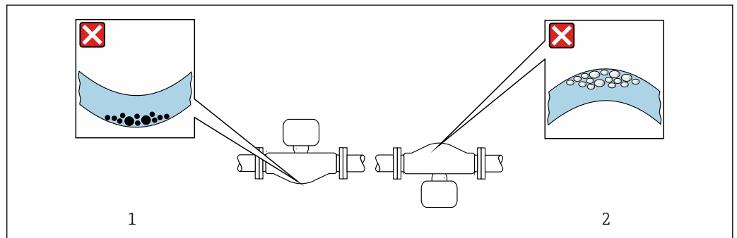
⑥ 弓形計測チューブセンサの取付方向
