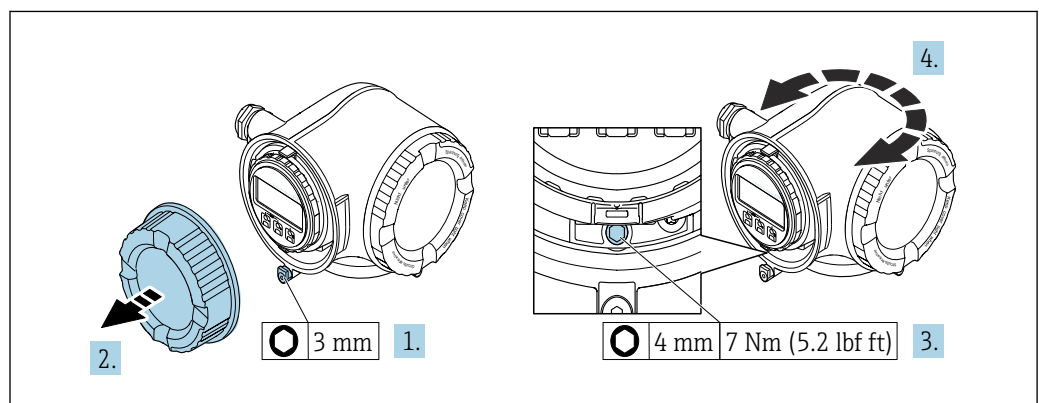
図 9 非防爆ハウジング
