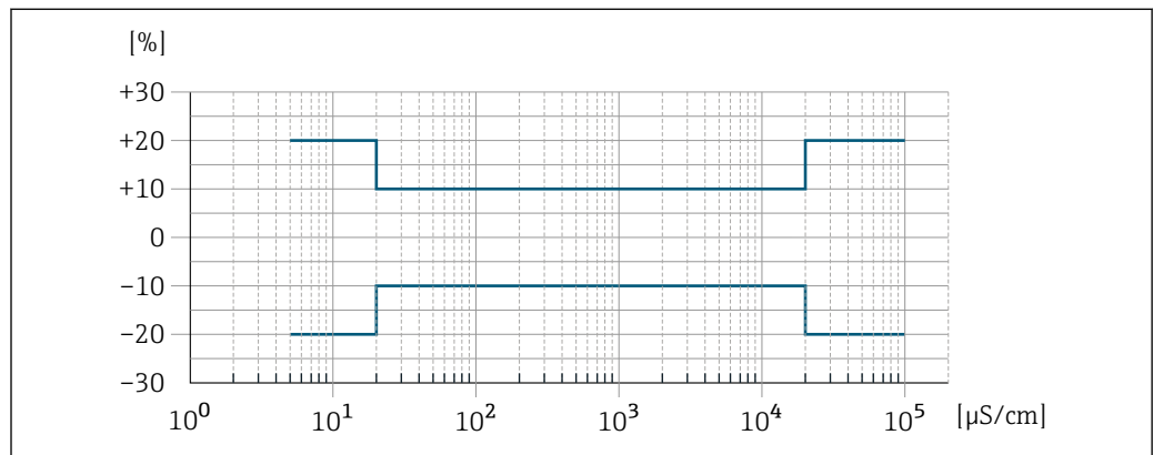
图 39 测量误差 (标准)
