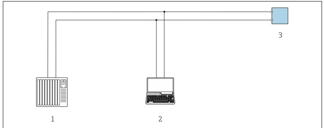
图 30 通过 Modbus RS485 通信进行远程操作（有源信号）
