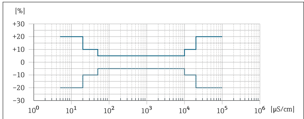
图 40 测量误差 (可选: 订购选项“电导率测量标定”, 选型代号 CW)
