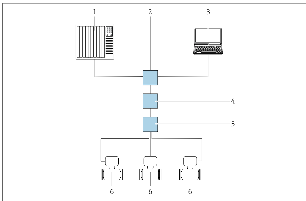
15 Opções para operação remota através do protocolo Modbus TCP por Ethernet-APL (ativa)
