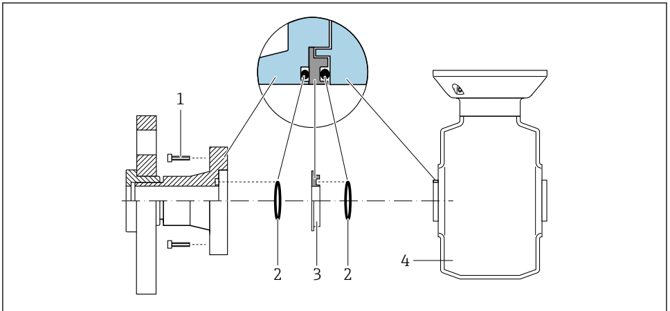
12 Földelőgyűrűk beépítése
